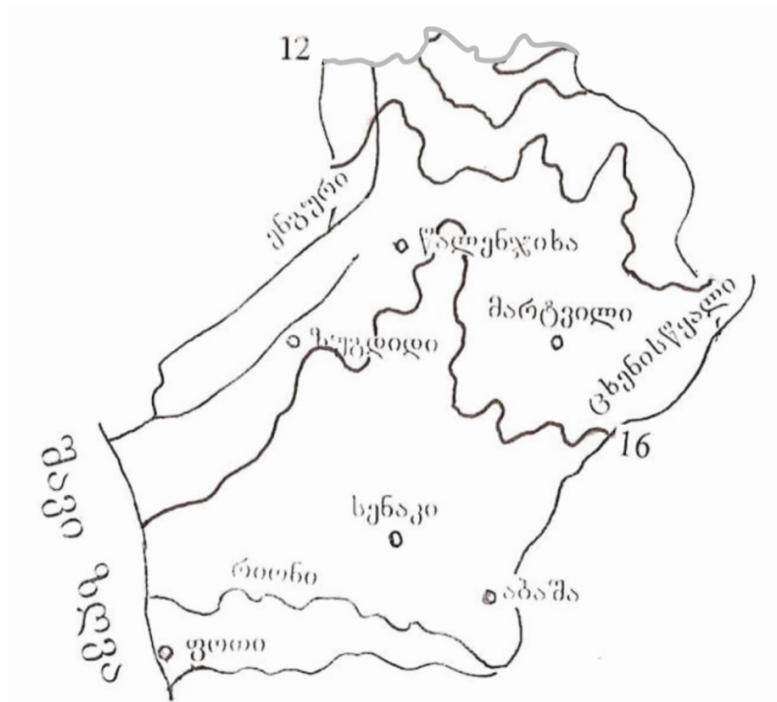
ნახ. 5. ჰაერის საშუალო თვიური ტემპერატურა. ოქტომბერი
