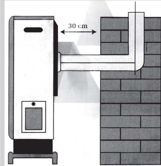
ყურადღებამ გამოთბობელი კედლიდან არანაკლებ 30 სმ-ით უნდა იყოს დაცილებული. გამოთბობლის საკვამლე მილი გარეთ გასვლისას 90 — გრადუსიან კუთხეს უნდა ქმნიდეს. საკვამლე მილის ბოლო ჭერის დანიდან 70 სმ-ით მაღლა უნდა იყოს. გამოთბობელზე არ შეიძლება ჩაიდნის შემოდგმა.
