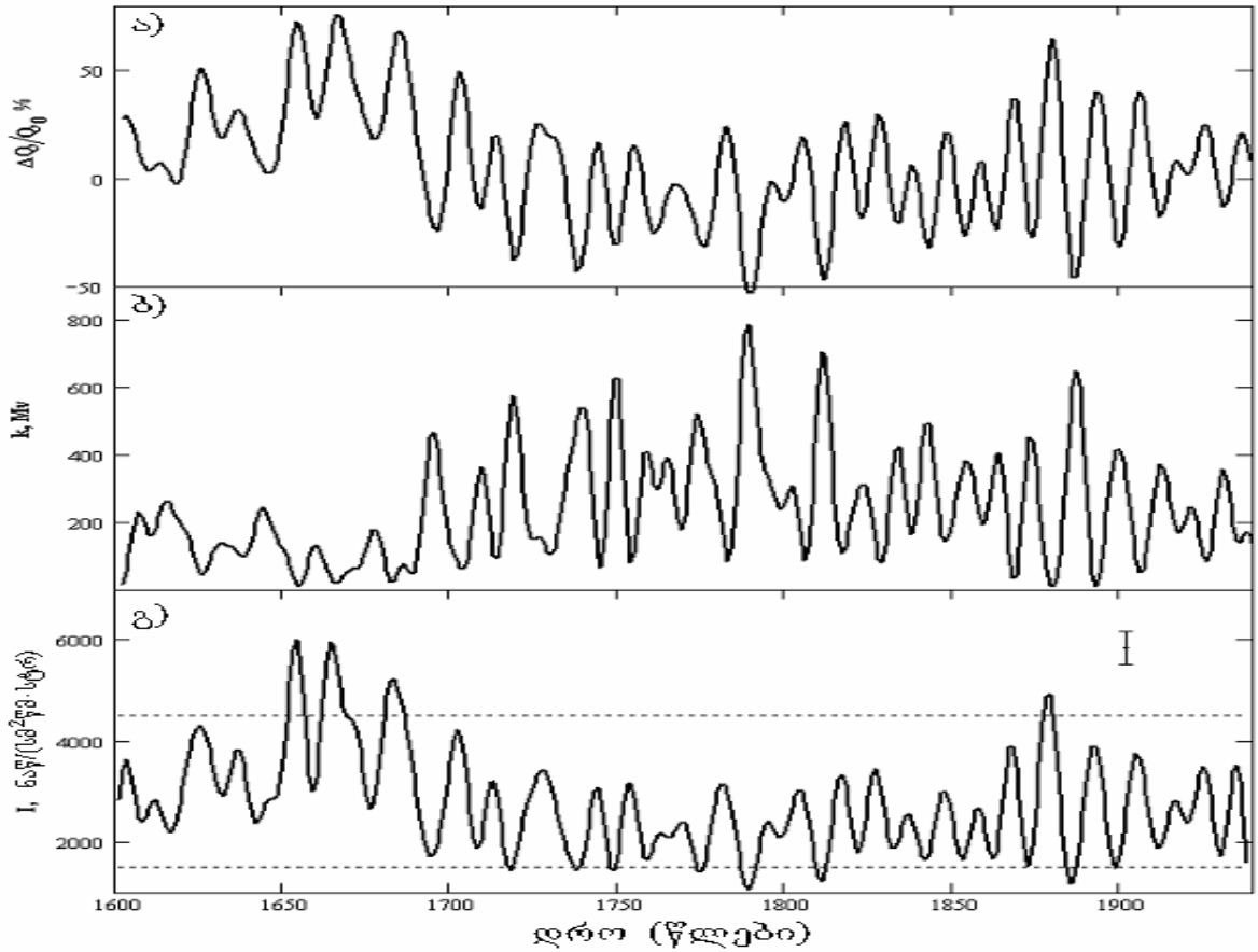
ნახ.48. ^{14}C –ის წარმოქმნის სიჩქარის (ა), მოდულაციის პარამეტრის (ბ) და კოსმოსური სხივების ინტენსივობის დროითი მრუდი (გ), 1600 – 1950 წლებში. გ) - ზე ტეხილი ხაზებით აღნიშნულია კოსმოსური სხივების ინტენსივობის ცვლილების დღეისათვის დაკვირვებადი ინტერვალი.
