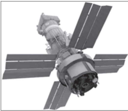
რადიოელექტრონული დაზვერვის რუსული სამხედრო კოსმოსური თანამგზავრი „კოსმონა“
