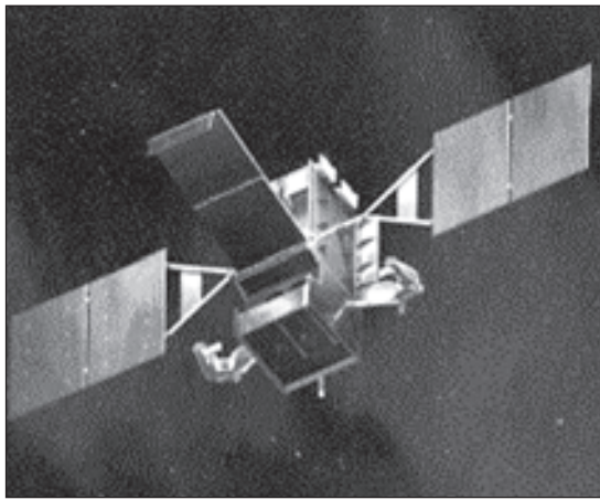
ამერიკული სადაზვერვო კოსმოსური თანამგზავრი USA241 (SBIRS-CE02).
