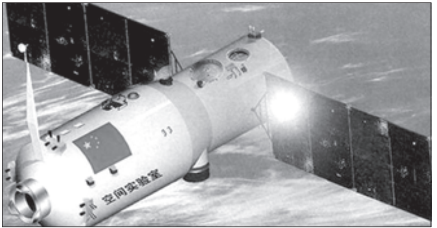
ჩინური კოსმოსური თანამგზავრი-ლაბორატორია „ტიანჰუი-2“.
