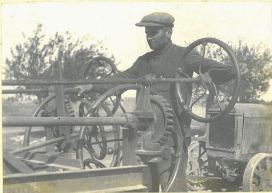
ГРЕЙДЕР ЗА РАБОТОЙ.
