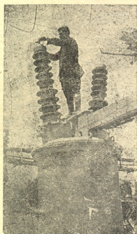
კასპის ელექტრო სადგურზე ისოლატორების მონტაჟი.
