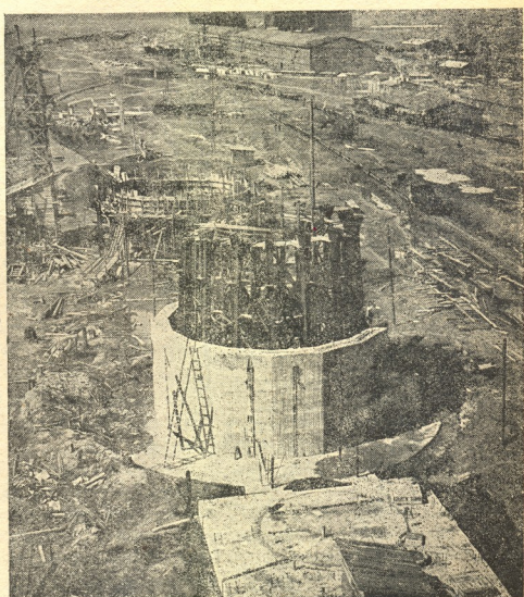
ჩელაბინსკის კარხნის მშენებლობაზე.
