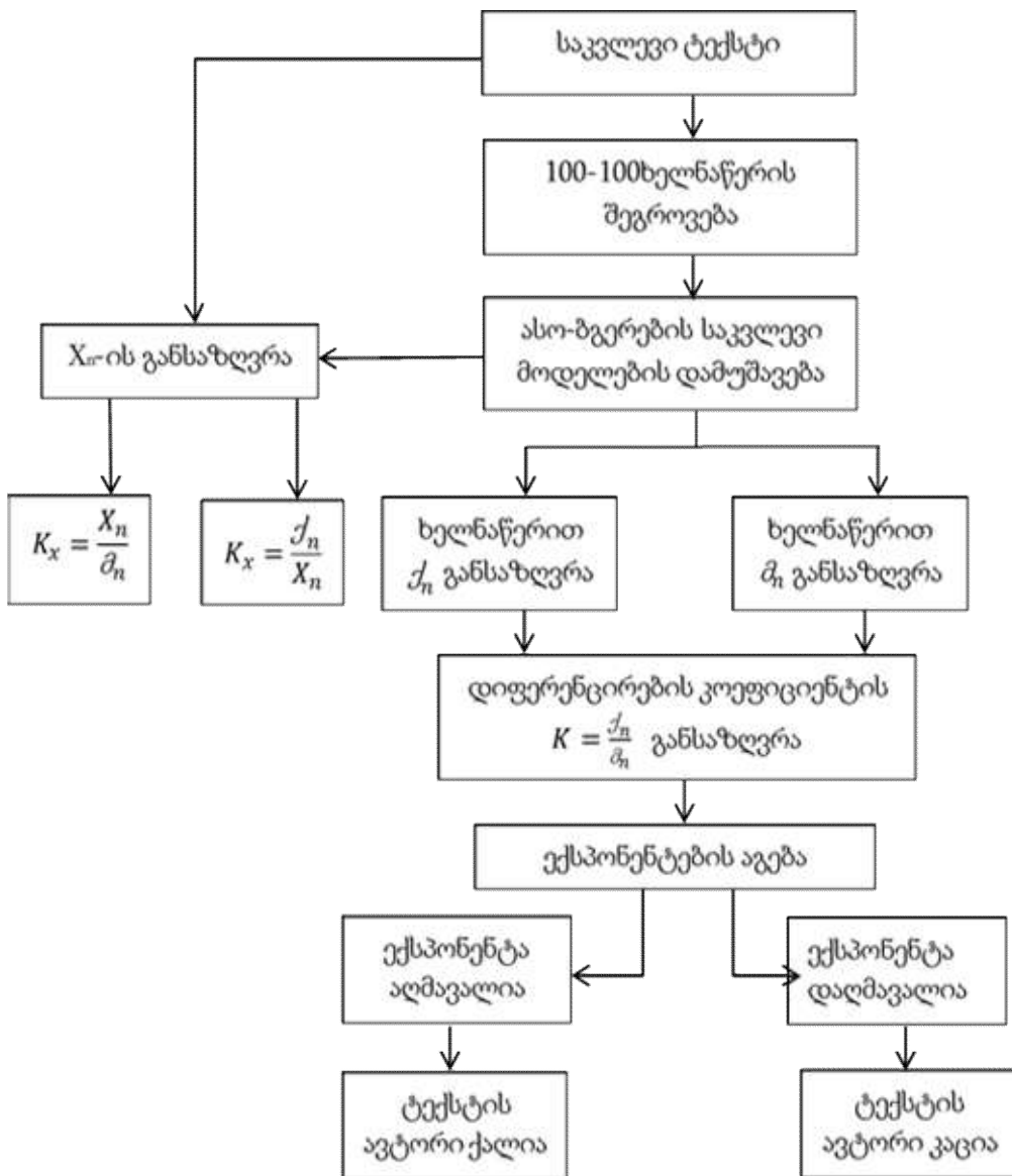
სურ.6. სქესის გამოცნობის ალგორითმი
