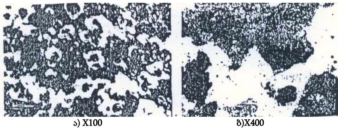
სურათი 1. სხმული თუჯი (C=3,3%; Si=2,75%.)
