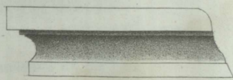
F. 9. Corniche Arménienne à Dilijan.
