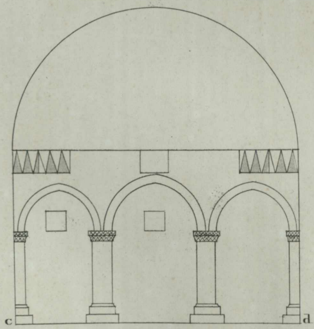
Coupe de l'Église ou Mosquée de cad
