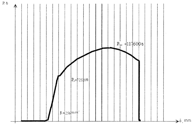
ნახ.9. შენადული ნაკერის გაჭიმვის დიაგრამა (III): ნიმუში №3.
