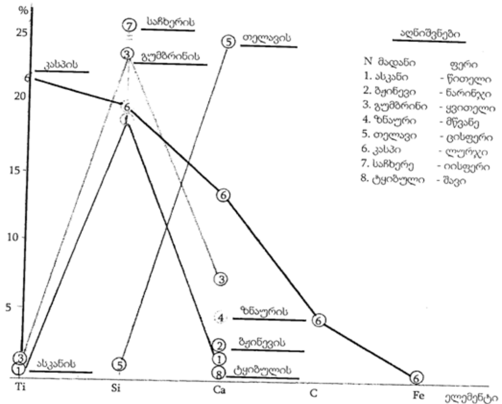
ნახ. 1. საქართველოს წიაღისეულთა შემადგენლობაში არსებული შედეგების ელექტროდის დანაფარში საჭირო ძირითად ელემენტთა რაოდენობრივი მაჩვენებლები
