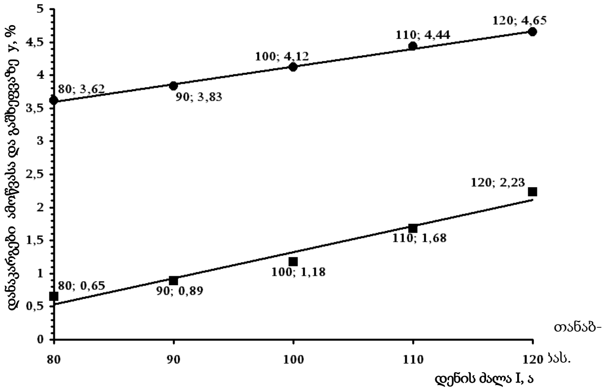
ნახ. 6. ამოწვასა და გაშხეფვაზე დასაკარგების დამოკიდებულება შედუღების დენის ძალაზე
