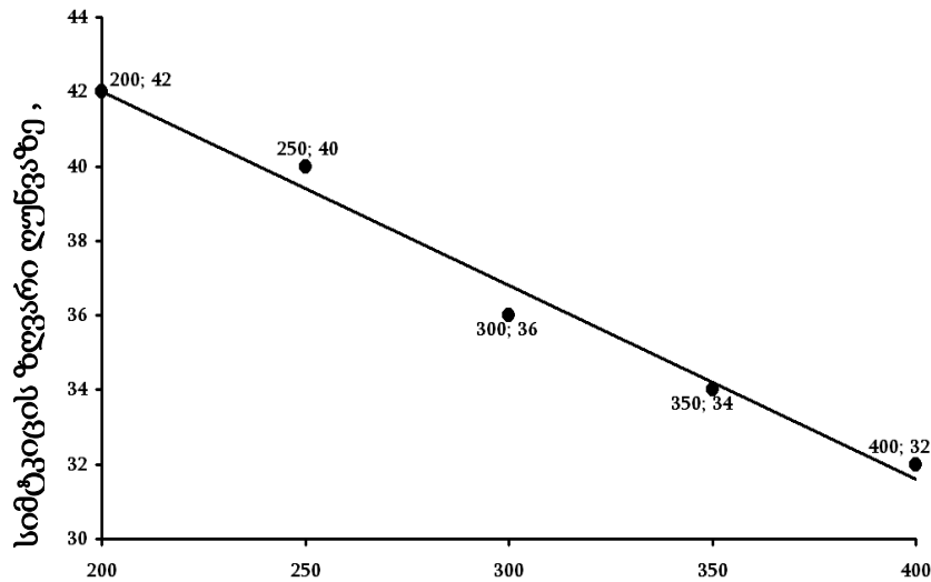
გამოწვის ტემპერატურა t_{\text{გამოწ.}}, \text{ }^{\circ}\text{C} ნახ.4. დანაფარის ღუნვაზე სიმტკიცის ზღვრის დამოკიდებულება ტემპერატურაზე.
