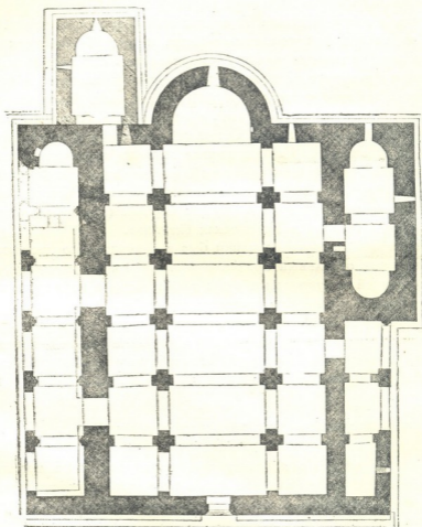
Рис. 1. План по обмеру арх. Цналы Г а б а ш в и л и 1936 года.
