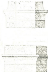
Рис. 87. Импосты арок на столбах по обмеру.
