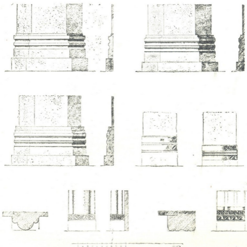
Рис. 86. Базы столбов и пилястр по обмеру
