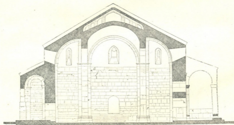
Рис. 5. Поперечный разрез с видом на восток.
