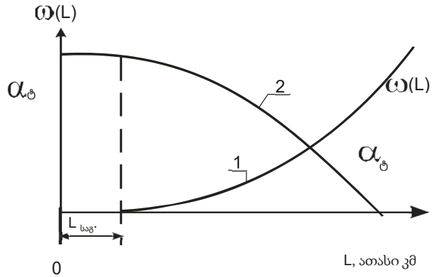
ნახ. 1. მტყუნებათა ნაკადის პარამეტრის \lambda(L) -1 და ტექნიკურად მზადყოფნის კოეფიციენტის კოეფიციენტის \alpha_{ტ} -2 ცვლილება ექსპლუატაციის მიხედვით.
