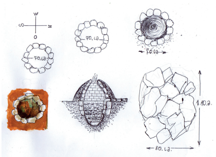
ჭოროხი, ჭარნალი, რკინის სადნობი ქურა-სახელოსნო, ძვ.წ. IX ს. Chorokhi, Charnali, steelmaking furnace, workshop, IX C. B.C.
