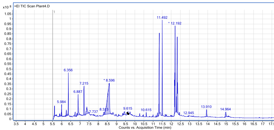
სურ. №65. ბათუმის ბოტანიკური ბაღის ცენტრალური პარკის ლოკაციაზე აღებული Polianthes tuberosa L. ბოლქვების ექსტრაქტის GC-MS ქრომატოგრამა.
