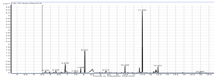
სურ. №5. ბათუმის ბოტანიკური ბაღის ავსტრალიის ფიტოგეოგრაფიული განყოფილების ლოკაციაზე აღებული Iris pallida Lam. ფესურების ექსტრაქტის GC-MS ქრომატოგრამა.
