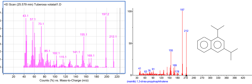
სურ. №7. 25,57 - 1,3-di-isopropylnaphthalene
