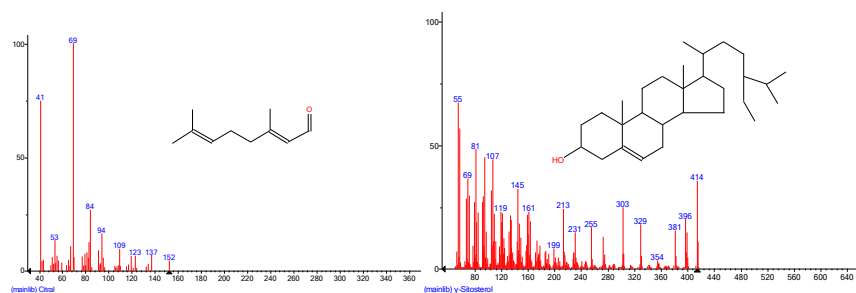
სურ. №3. ციტრალისა და გამა-სიტოსატეროლის მასსპექტრები
