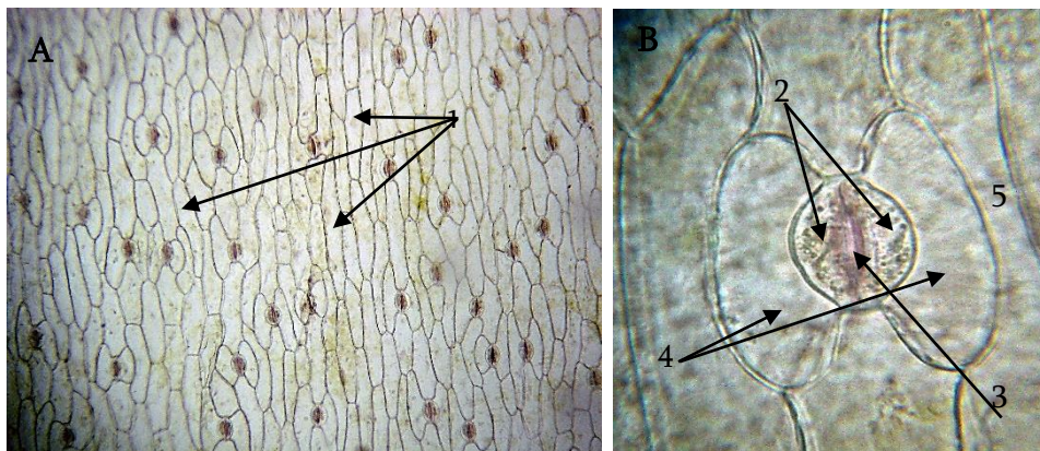
სურ. №45. Polianthes tuberosa L. - ს ფოთლის ეპიდერმისის მიკროსტრუქტურა: A. ფოთლის ეპიდერმისის ფუძემდებარე ქსოვილის პანორამა; B. ბაგის აპარატი; 1. არადაავირისტებული, სწორხაზოვანი, სათითურა-რომბისებური ტიპის უჯრედები; 2. ბაგის მკეტავი უჯრედები; 3. ბაგეთმორისი ხვრელი; 4. სატელიტი უჯრედები; 5. ქლოროპლასტები.
