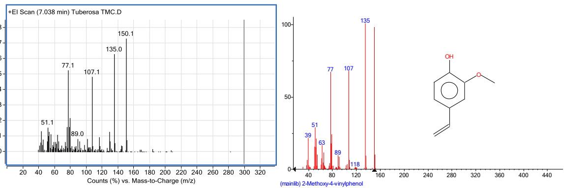
სურ. №18. 7,03 - p-Vinylguaicol: 2-Methoxy-4 vinylphenol
