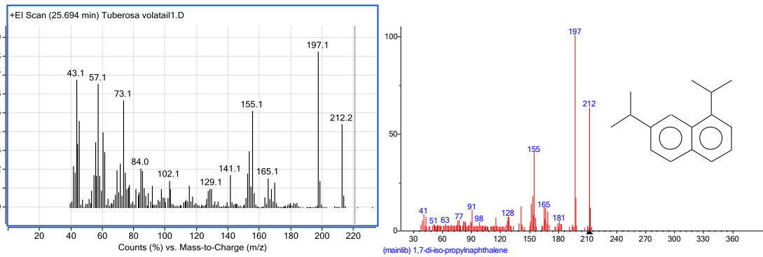
სურ. №8. 25,69 - 1,7-di-isopropylnaphthalene
