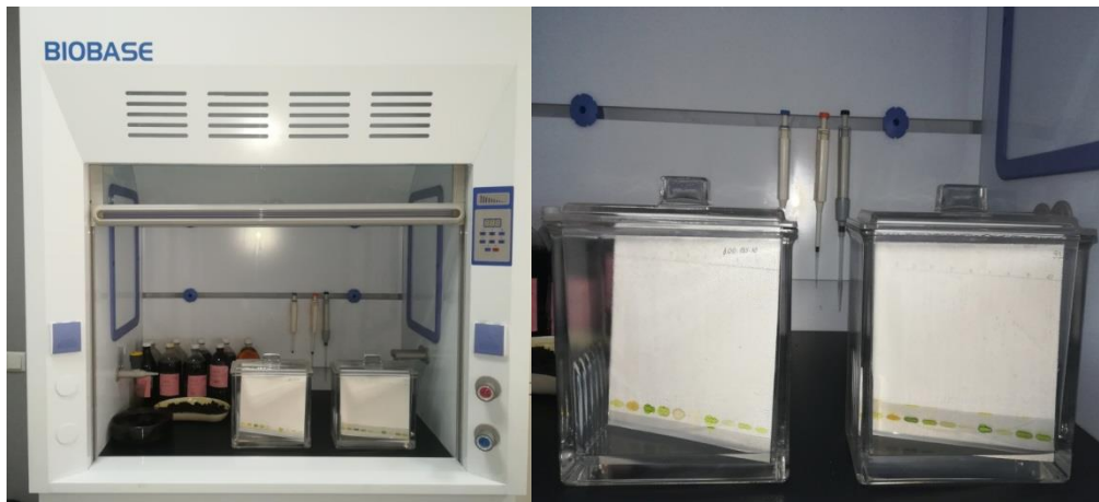
სურ. № 3. სილიკაგელის ქრომატოგრაფიული ფირფიტები გლიკოზიდების და აგლიკონების სისტემაში
