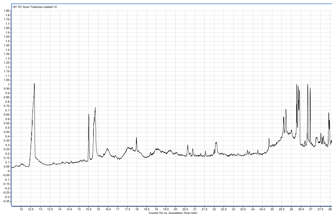
სურ. №1. Polianthes tuberosa L.-ს ყვავილების ექსტრაქტის GC-MS ქრომატოგრამა
