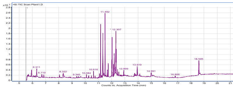
სურ. №1. ბათუმის ბოტანიკური ბაღის არომატულ მცენარეთა ექსპერიმენტულ ნაკვეთზე აღებული Polianthes tuberosa L. ბოლქვების ექსტრაქტის GC-MS ქრომატოგრამა.
