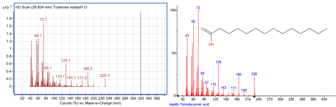
სურ. №9. 26,82 - Myristic acid.
