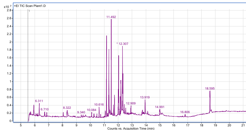
სურ. №62. ბათუმის ბოტანიკური ბაღის არომატულ მცენარეთა ექსპერიმენტულ ნაკვეთზე აღებული Polianthes tuberosa L. ბოლქვების ექსტრაქტის GC-MS ქრომატოგრამა.
