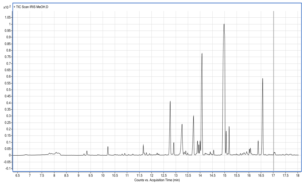
სურ. №70. Iris pallida Lam.-ს ფესურებისგან „მწვანე ტექნოლოგიებით“ მიღებული ეთერზეთის GC-MS ქრომატოგრამები.
