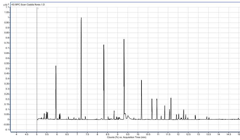
სურ. №7. Cassia angustifolia - ს ყვავილების ექსტრაქტის GC-MS ქრომატოგრამა
