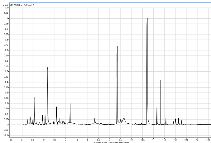
სურ. №4. Coffea Arabica - ს ფოთლების ექსტრაქტის GC-MS ქრომატოგრამა
