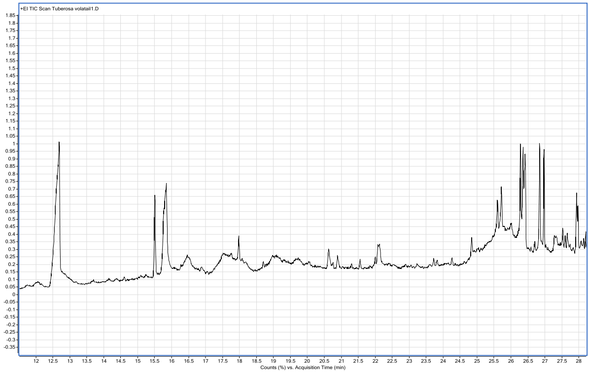
სურ. №60. Polianthes tuberosa L.-ს ყვავილების ექსტრაქტის GC-MS ქრომატოგრამა.
