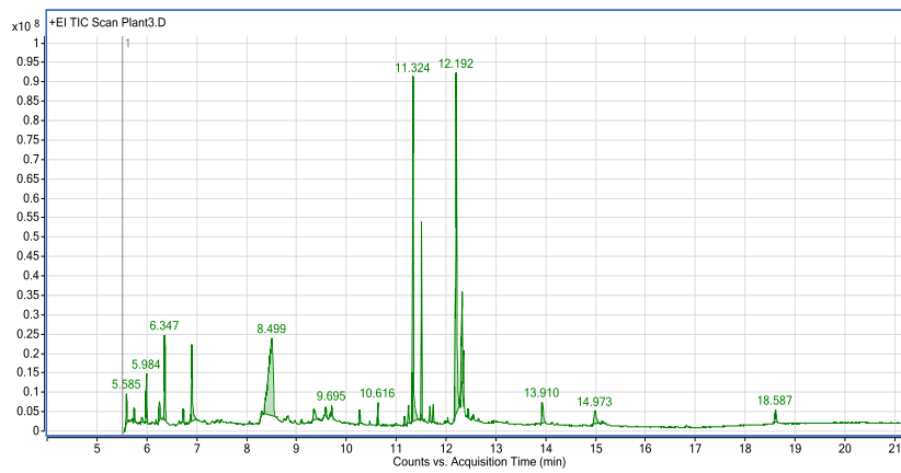
სურ. №64. ბათუმის ბოტანიკური ბაღის ავსტრალიის ფიტოგეოგრაფიული განყოფილების ლოკაციაზე აღებული Polianthes tuberosa L. ბოლქვების ექსტრაქტის GC-MS ქრომატოგრამა.
