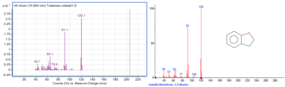
სურ. №3. 15,5 - Coumaran: 2,3 - DihydroBenzofuran
