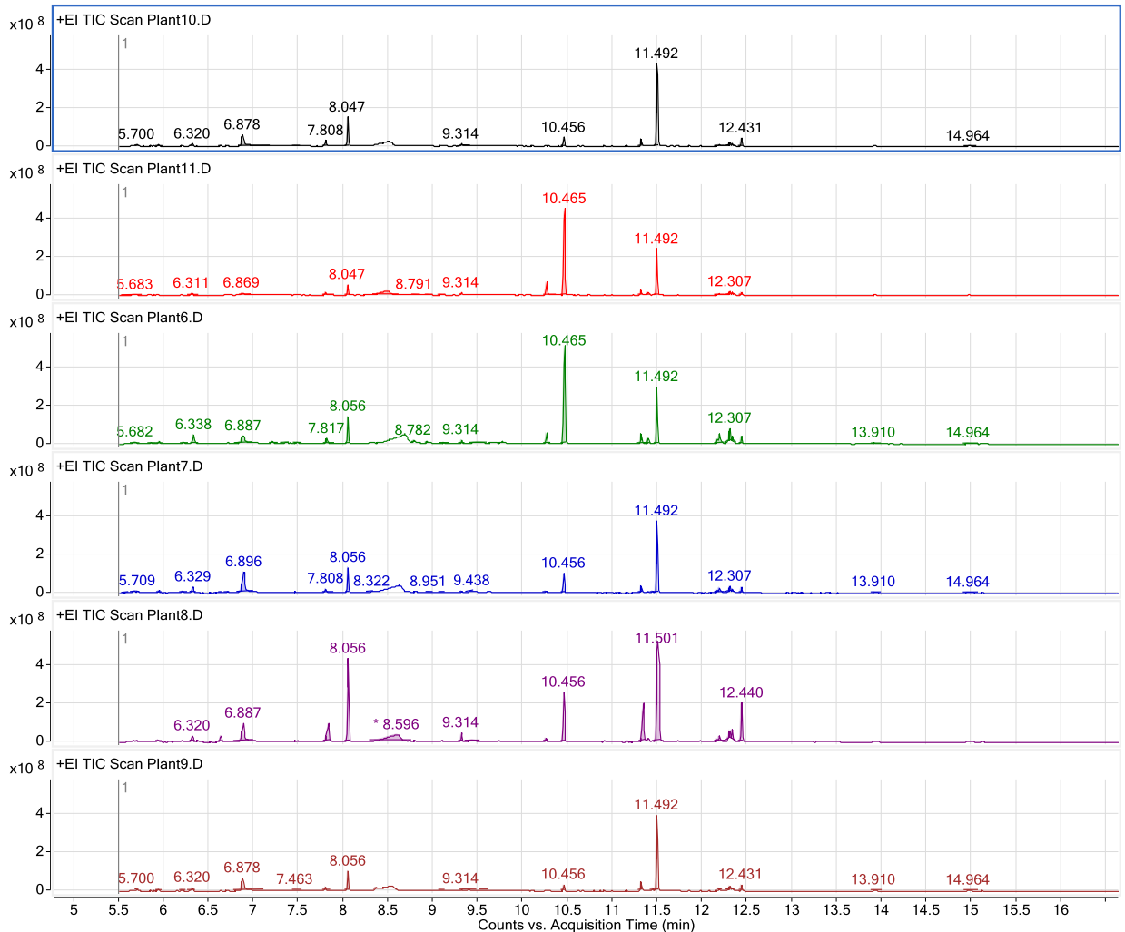
სურ. №68. ბათუმის ბოტანიკური ბაღის ექვსი ლოკაციიდან აღებული Iris pallida Lam.-ს ფესურების GC-MS ქრომატოგრამები.
