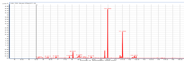
სურ. №6. ბათუმის ბოტანიკური ბაღის არომატულ მცენარეთა ექსპერიმენტული ნაკვეთის ლოკაციაზე აღებული Iris pallida Lam. ფესურების ექსტრაქტის GC-MS ქრომატოგრამა.
