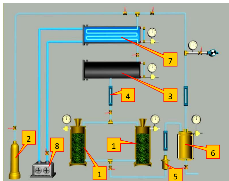
სურათი №1. გათხევადებული აირით ექსტრაქციის დანადგარი.
