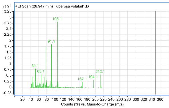
სურ. №10. 26,94 - Benzyl Benzoate
