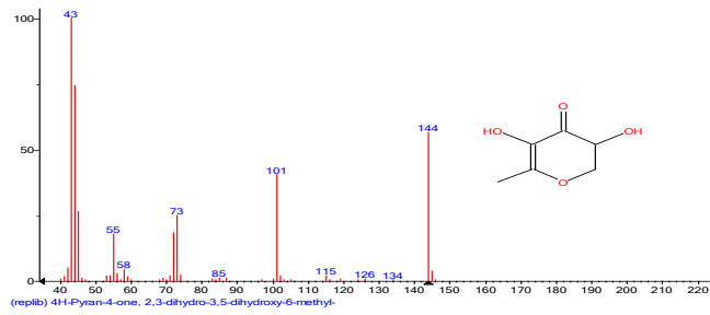
სურ. №8. 2,3-დიჰიდრო-3,5-დიჰიდროქსი-6-მეთილ-4H - პირან-4-ონის მასსპექტრი
