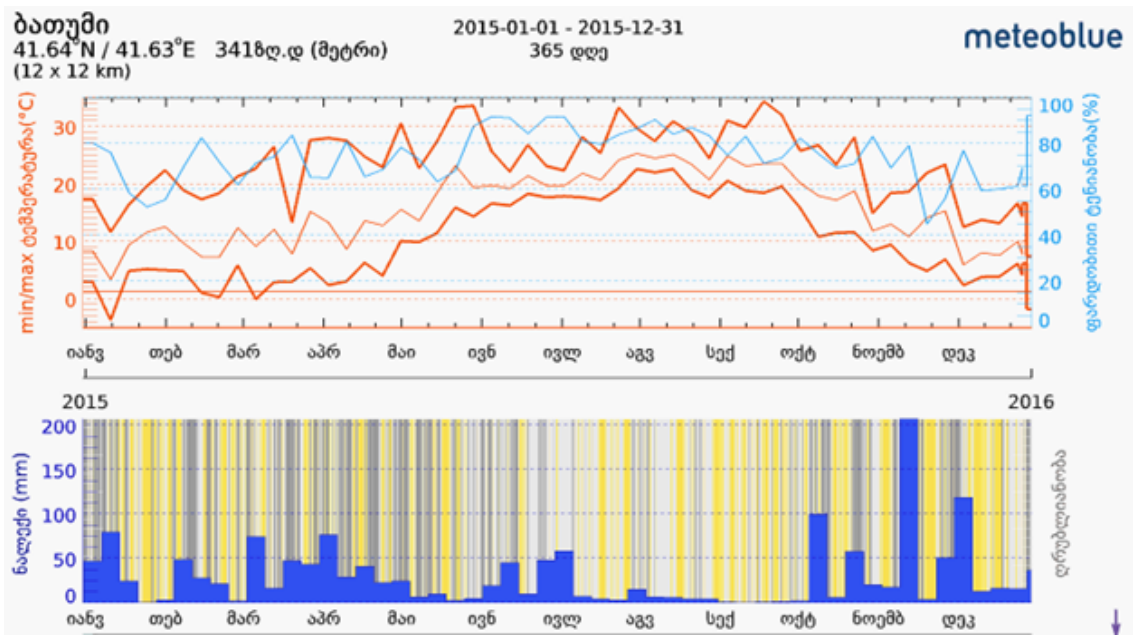
სურ .№2. ბათუმის ზღვის სანაპიროს 2015 წლის მეტეოროლოგიური მონაცემები.
