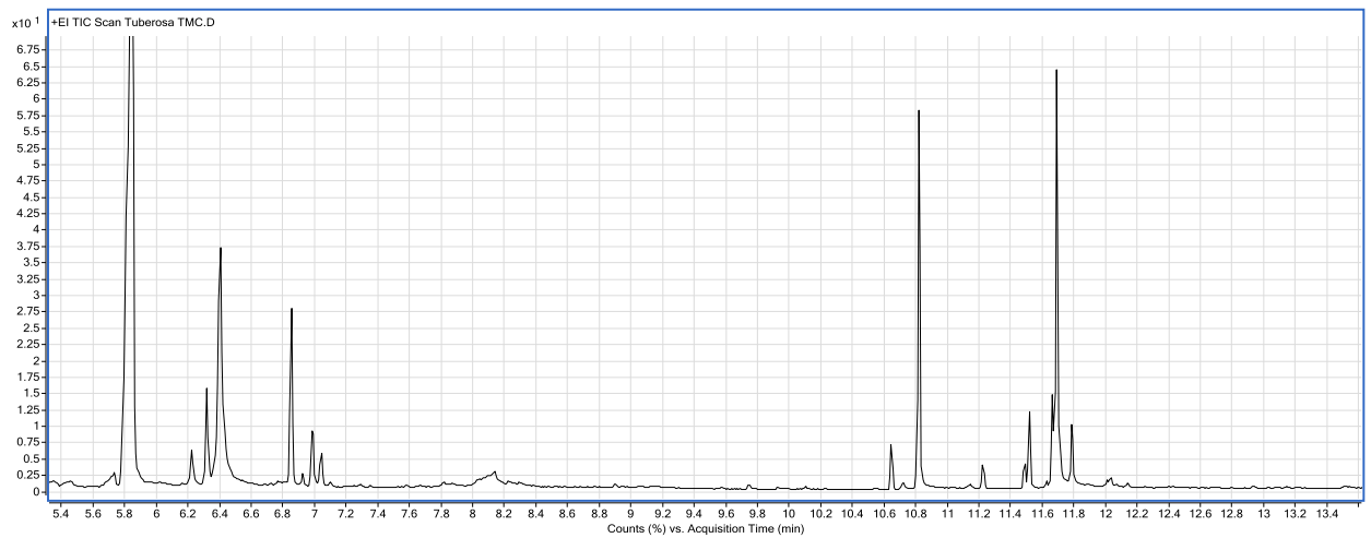
სურ. №61. Polianthes tuberosa L.-ს ყვავილების ექსტრაქტის GC-MS ქრომატოგრამა.
