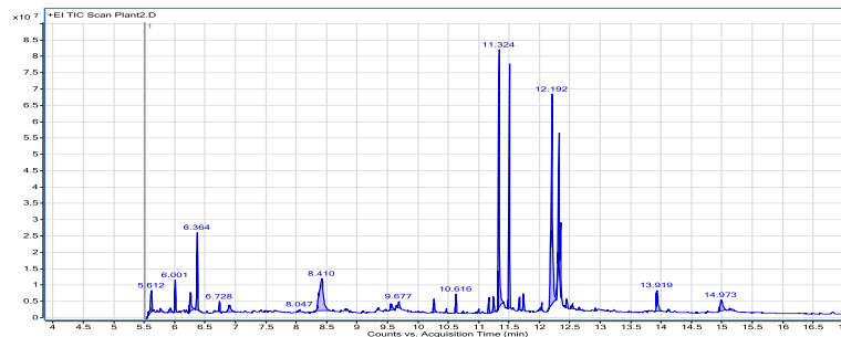
სურ. №2. ბათუმის ბოტანიკური ბაღის ჰიმალაის ფიტოგეოგრაფიული განყოფილების ლოკაციაზე აღებული Polianthes tuberosa L. ბოლქვების ექსტრაქტის GC-MS ქრომატოგრამა.
