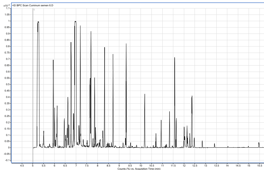
სურ. №69. Cuminum cyminum L. - ის თესლების GC-MS ქრომატოგრამა.
