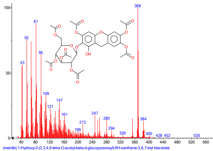
სურ. №8. 1- ჰიდროქსი-2 (2,3,4,6 - ტეტრა - O - აცეტილ - ბეტა - d - გლუკოპირანოზილ) 9H - ქსანტენ-3,6,7-ტრიილ ტრიაცეტატის მასსპექტრი
