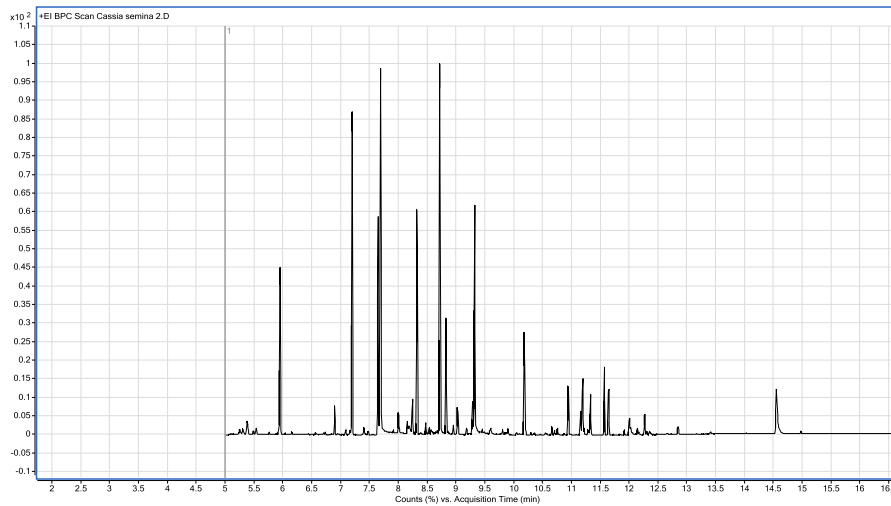
სურ. №5. Cassia angustifolia - ს თესლების ექსტრაქტის GC-MS ქრომატოგრამა
