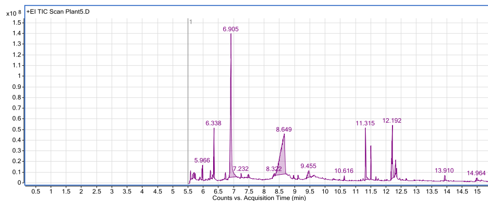
სურ. №66. ბათუმის ბოტანიკური ბაღის ევროპის ფიტოგეოგრაფიული განყოფილების ლოკაციაზე აღებული Polianthes tuberosa L. ბოლქვების ექსტრაქტის GC-MS ქრომატოგრამა.
