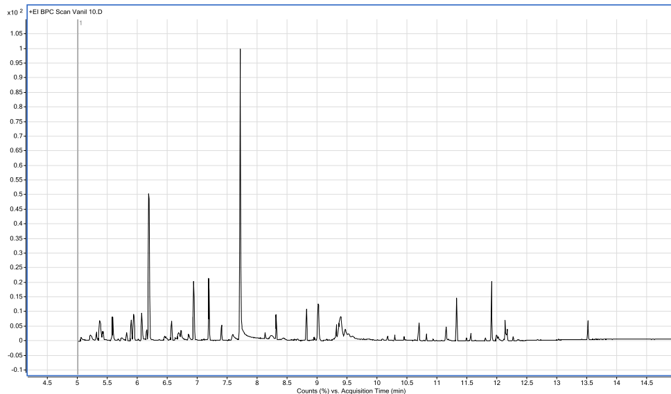
სურ. № 1. Vanilla planifolia - ს ფოთლების ექსტრაქტის GC-MS ქრომატოგრამა
