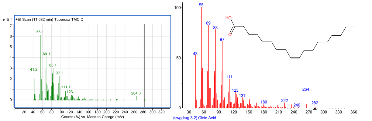
სურ. №22. 11,68 - Oleic Acid
