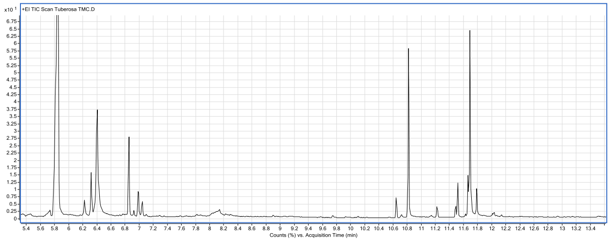
სურ. №14. Polianthes tuberosa L.-ს ყვავილების ექსტრაქტის GC-MS ქრომატოგრამა
