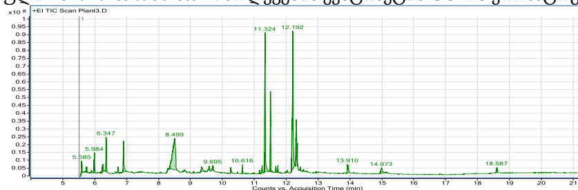
სურ. №2. ბათუმის ბოტანიკური ბაღის ჰიმალაის ფიტოგეოგრაფიული განყოფილების ლოკაციაზე აღებული Polianthes tuberosa L. ბოლქვების ექსტრაქტის GC-MS ქრომატოგრამა.
