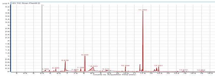
სურ. №4. ბათუმის ბოტანიკური ბაღის ჩრდილოეთ ამერიკის ფიტოგეოგრაფიული განყოფილების ლოკაციაზე აღებული Iris pallida Lam. ფესურების ექსტრაქტის GC-MS ქრომატოგრამა.
