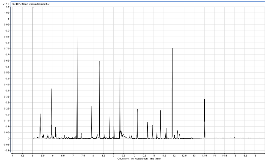
სურ. №6. Cassia angustifolia - ს ფოთლების ექსტრაქტის GC-MS ქრომატოგრამა
