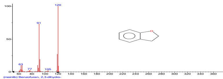
სურ. №2. დიჰიდრობენზოფურანის მასსპექტრი
