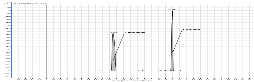
სურ. №71. Cuminum cyminum L.-ს თესლებისგან „მწვანე ტექნოლოგიებით“ მიღებული ეთერზეთის GC-MS ქრომატოგრამები.
