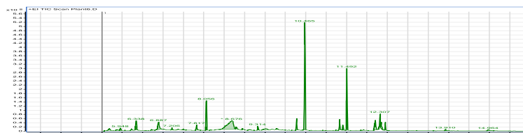
სურ. №8. ბათუმის ბოტანიკური ბაღის ცენტრალური პარკის ლოკაციაზე აღებული Iris pallida Lam. ფესურების ექსტრაქტის GC-MS ქრომატოგრამა.
