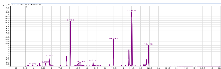
სურ. №1. ბათუმის ბოტანიკური ბაღის ჰიმალაის ფიტოგეოგრაფიული განყოფილების ლოკაციაზე აღებული Iris pallida Lam. ფესურების ექსტრაქტის GC-MS ქრომატოგრამა.
