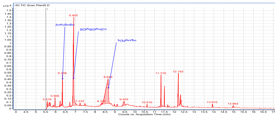
სურ. №6. ბათუმის ბოტანიკური ბაღის ევროპის ფიტოგეოგრაფიული განყოფილების ლოკაციაზე აღებული Polianthes tuberosa L. ბოლქვების ექსტრაქტის GC-MS ქრომატოგრამა.
