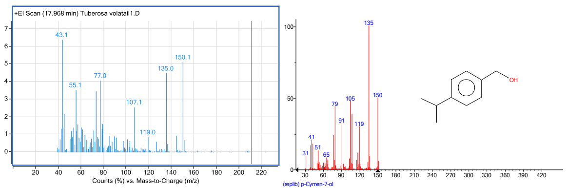
სურ. №5. 17,96 - p-Cymen-7-ol
