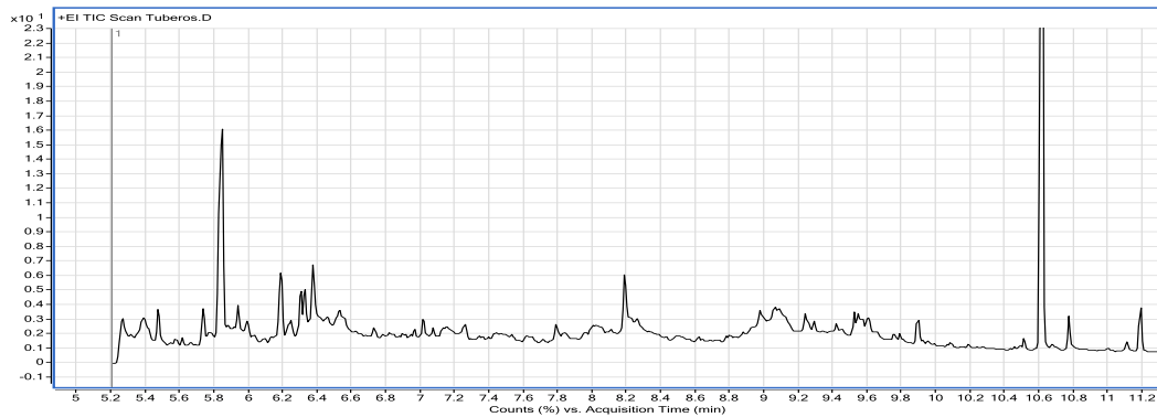
სურ. №72. Polianthes tuberosa L. ყვავილებისგან „მწვანე ტექნოლოგიებით“ მიღებული ეთერზეთის GC-MS ქრომატოგრამები.
