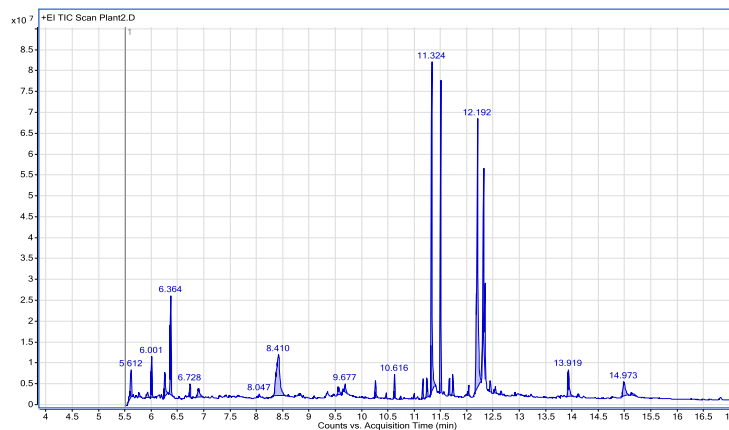
სურ. №63. ბათუმის ბოტანიკური ბაღის ჰიმალაის ფიტოგეოგრაფიული განყოფილების ლოკაციაზე აღებული Polianthes tuberosa L. ბოლქვების ექსტრაქტის GC-MS ქრომატოგრამა.
