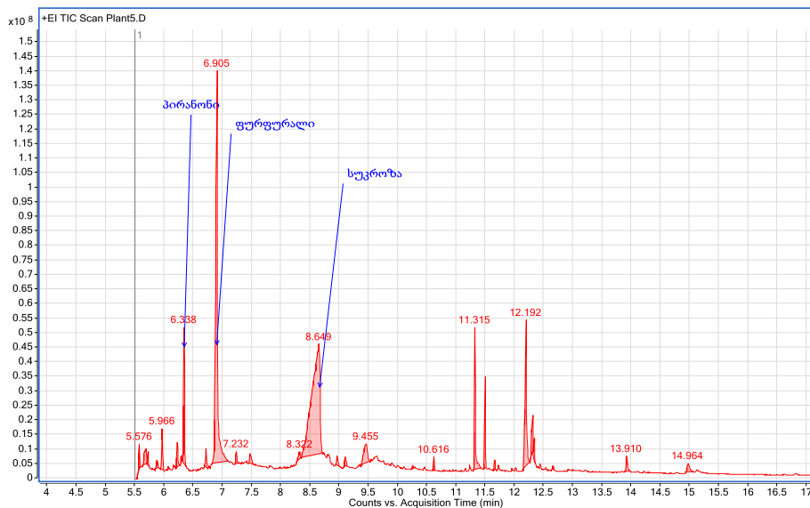
სურ. № 67. ბათუმის ბოტანიკური ბაღის ევროპის ფიტოგეოგრაფიული განყოფილების ლოკაციაზე აღებული Polianthes tuberosa L. ბოლქვების ექსტრაქტის GC-MS ქრომატოგრამა, გამოკვეთილი დომინანტი ნივთიერებებით.
