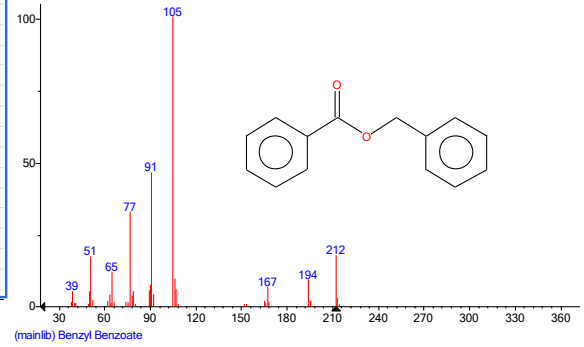
სურ. №10. 26,94 - Benzyl Benzoate
