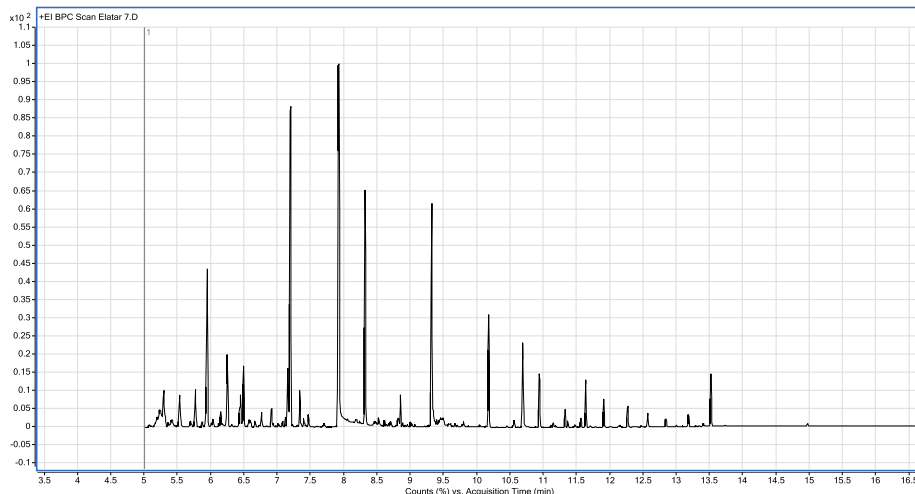
სურ. №2. Elletaria cardamomum - ის ფოთლების ექსტრაქტის GC-MS ქრომატოგრამა
