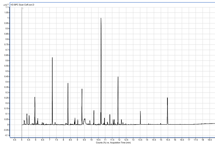
სურ. № 3. Coffea canephora - ს ფოთლების ექსტრაქტის GC-MS ქრომატოგრამა
