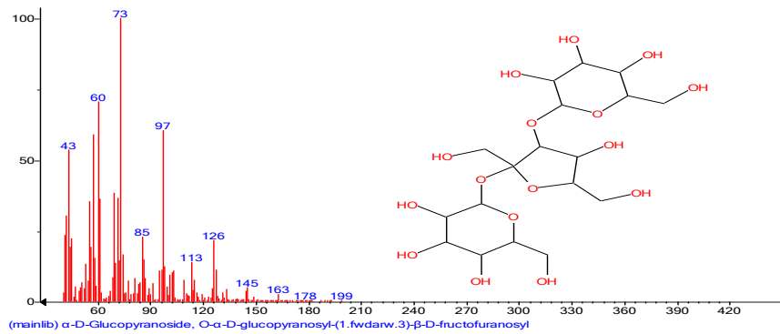
სურ. №10. მელეზიტოზის მასსპექტრი
