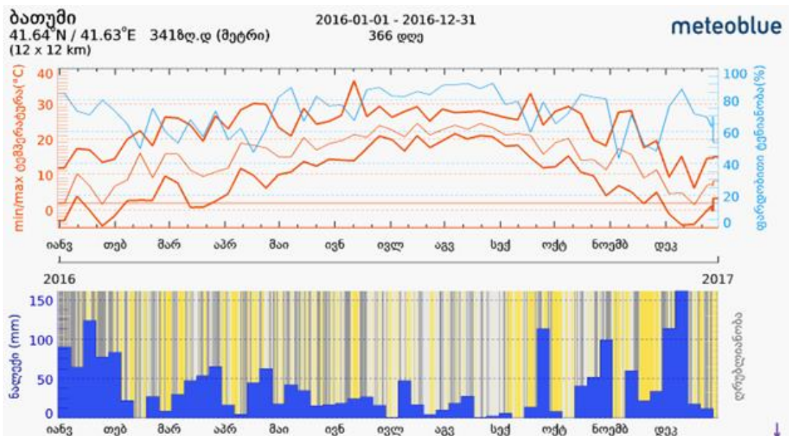
სურ. №3. ბათუმის ზღვის სანაპიროს 2016 წლის მეტეოროლოგიური მონაცემები.
