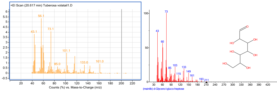
სურ. №6. 20,61 - d-Glycero-l-gluco-heptose
