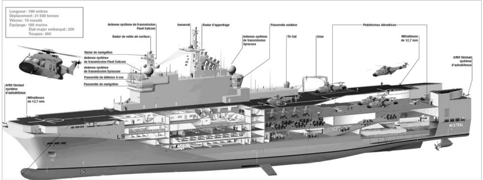
მინსტრალის კლასის გემის სქემა
