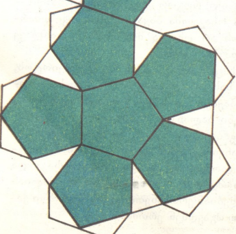
დოდეკაედრი
