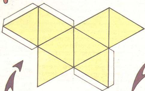
ოქტაედრი
