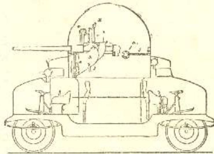
აეროპლანების სადევნი და დასახვრეტი ჯავშიანი ავტომობილის შინაგანი მოწყობილობა და მათი სასროლი ყუმბარები.
