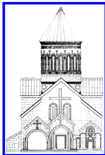
უკლათი. შასველეთის ფასადი
