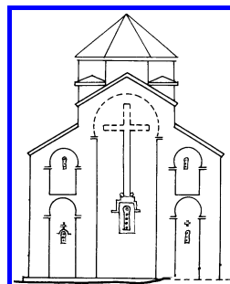
ურჯანის. ყველაწმინდის ეკლესია (VIII ს.). შასველის ფასადი
