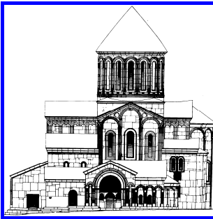
უკლათი. სამხრეთის ფასადი
