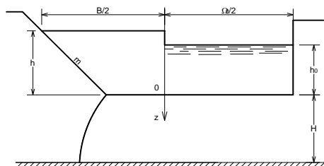
ნახ. 2 არხის განიკვეთის საანგარიშო სქემა
