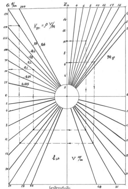
ნახ. 2. დატვირთვის სამუშაოების მწარმოებლურობის განსაზღვრა
