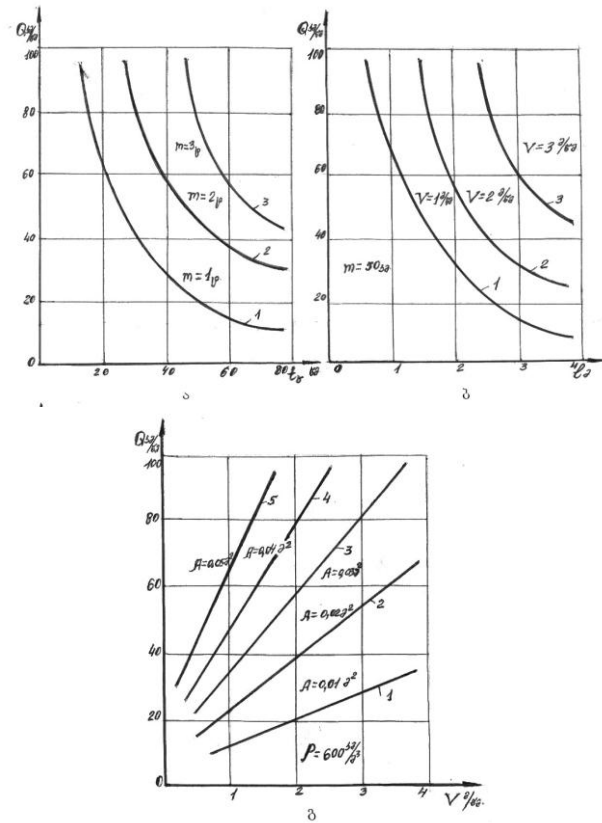
ნახ. 1. მწარმოებლურობის დამოკიდებულება ძირითად პარამეტრებზე
