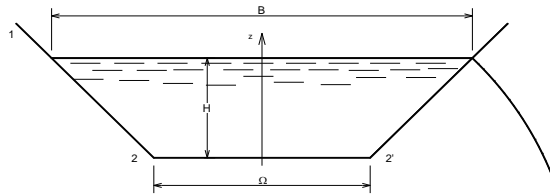
ნახ. №1. არხის ფილტრაციის საანგარიშო სქემა
