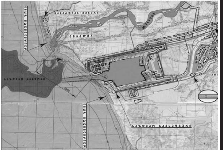
ანაკლიის სამომავლო პორტის ერთ-ერთი სქემატური მოდელი
