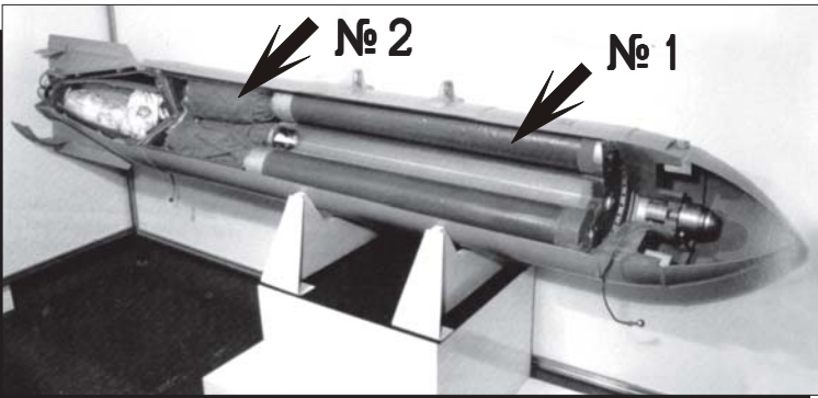
სტენდზე წარმოდგენილი CA5-250T-ის ქრილი. ისრებით მითითებულია №1 — მანათობელი ღერო და №2 — დაკეცილი პარაშუტი
