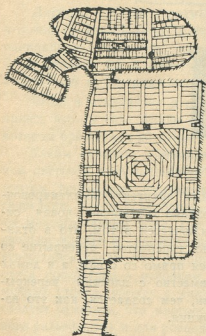
Рис. 2. Дарбази в селе Чачкари близ Вардзния. План (обмер Л. Сумбадзе), фасад и интерьер с натуры (фото арх. В. Гагошидзе).
