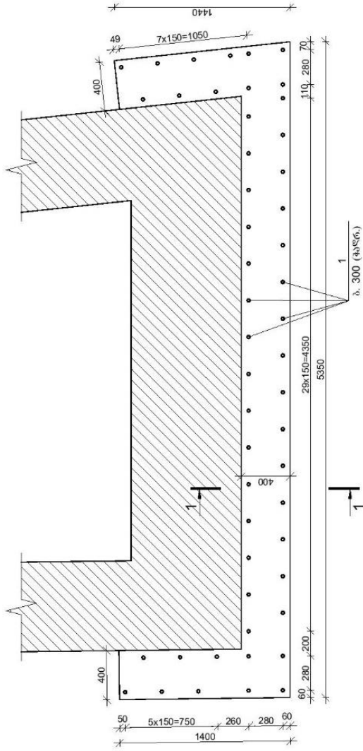
ანკერების განლაგების გეგმა
