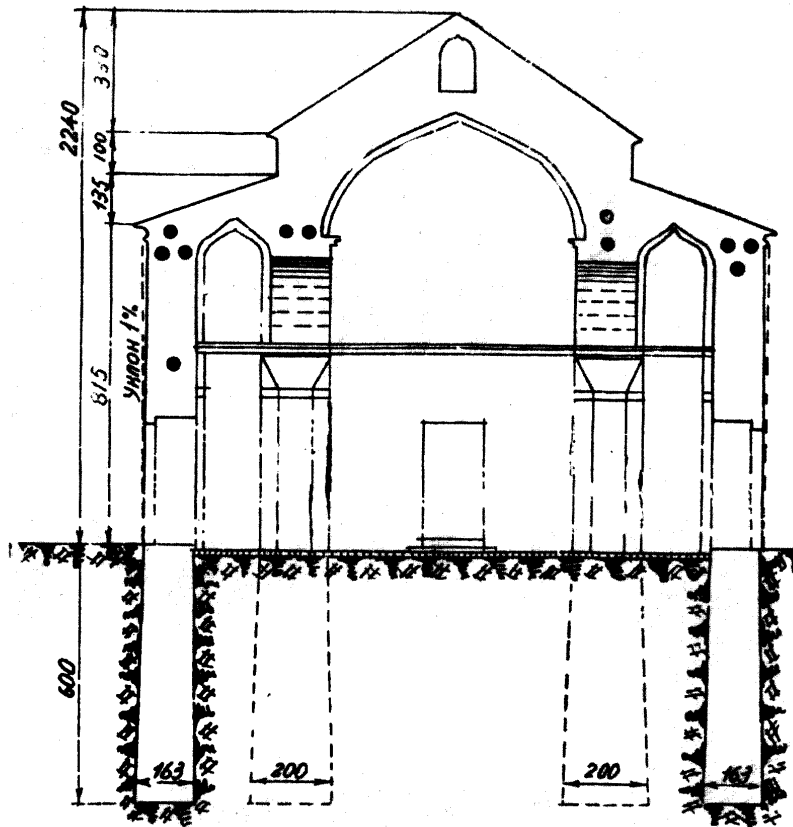
13. ჯიგრაშენის განივი ჭრილი სქემა.
