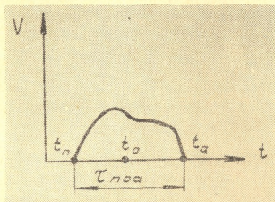
Рис. 5. Проектируемые, оптимальные в данных условиях, кривая скорости V и длительность \tau_{ноа} обслуживания в системе рисунка 4 объекта O_1 машиной M_2 при одном ее рейсе.
