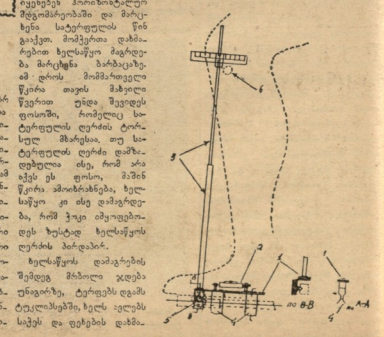
ბ. აბიძის, კავშირის მუშაობის სქემა
