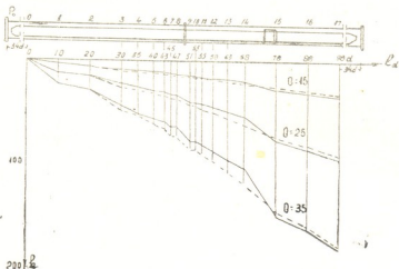
ნახ. 4. მილის სიგრძეზე დაწნევა h -ის ცვლილება სითხის სხვადასხვა ბარჯისას, როცა საკეტი მოთავსებულია გასასვლელში
