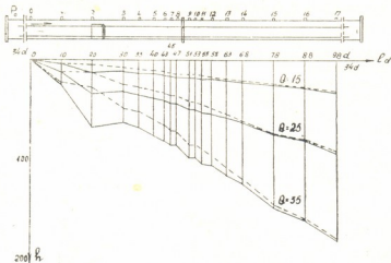
ნახ. 2. მილის სიგრძეზე დაწნევა h -ის ცვლილება სითხის სხვადასხვა, ხარჯისას, როცა რგოლურ სივრცეში საკეტი მოთავსებულია შესა- სვლელში: h — ვერცხლისწყლის სვეტის სიმაღლე მმ-ით
