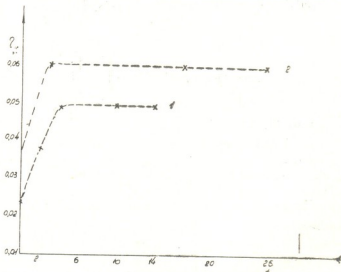
Рис. 1. Изменение удельной вязкости в процессе поликонденсации: 1— \alpha, \omega -дигидроксиметилфенилсилоксан + бис-(8-оксихинолин)дибутокситан ( n=6 ); 2— \alpha, \omega -дигидроксиметилфенилсилоксан + бис-(8-оксихинолин)дибутокситан ( n=11 )
