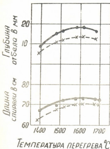
Рис. 4. Влияние перегрева на литейные свойства чугуна
