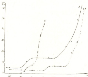
Рис. 2. Термомеханические кривые полимеров: 1— n=6 ; 2— n=11 ; 3— n=25
