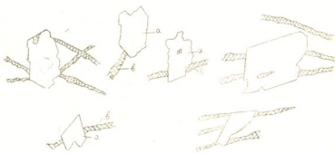
Рис. 5. Кристаллики альбита не пересекаются прожилками кальцита: а — альбит; б — кальцит
