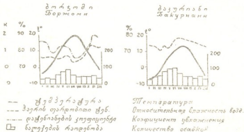
სურ. 1. ძირითადი მეტეოროლოგიური ელემენტების წლიური მსვლელობა ბორჯომ-ბაკურიანში (მ. კორძაბიას მიხედვით)
