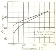
Рис. 1. Зависимость электросопротивления жидкого чугуна от температуры перегрева
