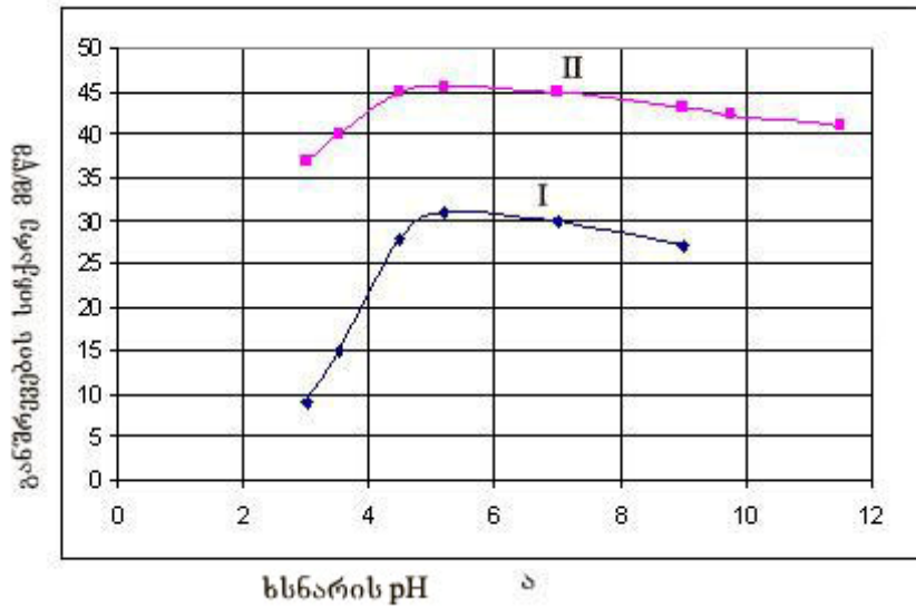
ნახ. 7. რეალურ ხსნარში განშრევების სიჩქარის ხსნარის pH-ზე დამოკიდებულება დამლექი: I- კალციუმის ჰიდროჟენგი; II - ნატრიუმის სულფიდი
