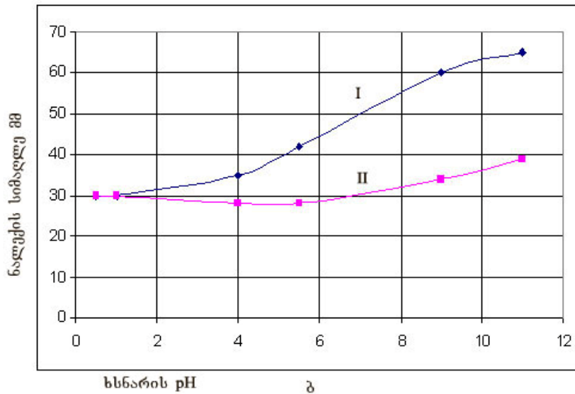
ნახ. 8 რეალურ ხსნარში გამოყოფილი ნალექების მოცულობის ხსნარის pH-ზე დამოკიდებულება. დამლექი: I- კალციუმის ჰიდროჟენგი; II- ნატრიუმის სულფიდი
