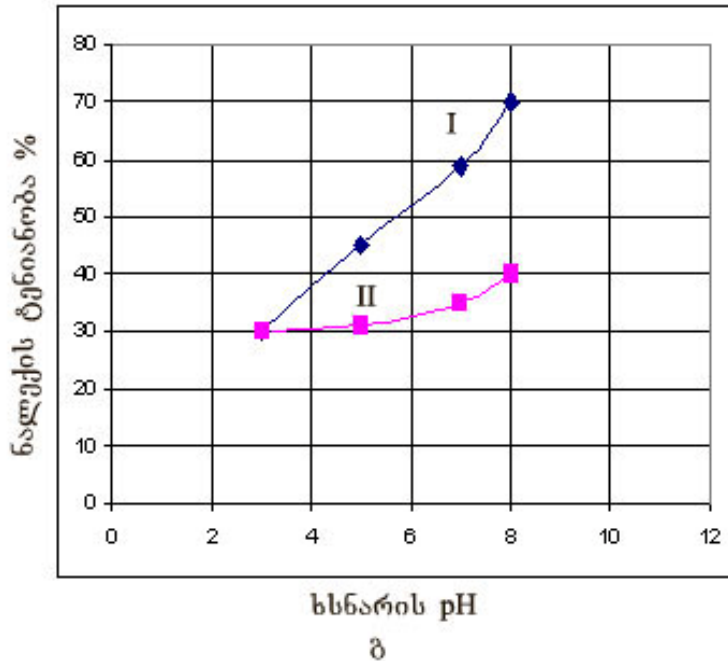
ნახ. 9. რეალურ ხსნარში გამოყოფილი ნალექების ტენიანობის ხსნარის pH-ზე დამოკიდებულება. დამლევი: I- კალციუმის ჰიდროჟანგი; II- ნატრიუმის სულფიდი
