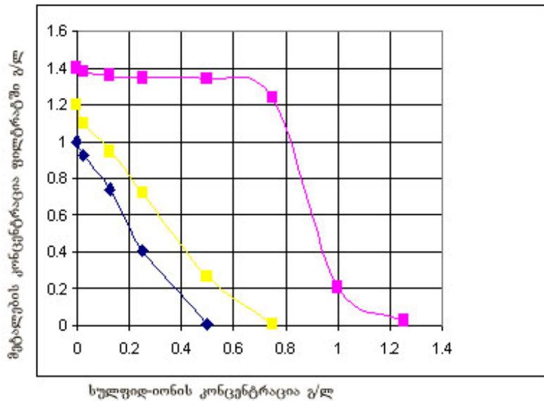
ნახ. 5 ხსნარში მეტალების იონების კონცენტრაციის დამოკიდებულება შეყვანილი სულფიდ-იონის რაოდენობაზე ■ Fe; ■ Zn; ■ Cu
