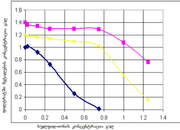
ნახ. 6 ნარევი ინდივიდუალური მეტალის იონების კონცენტრაციის შეყვანილი სულფიდ-იონის რაოდენობაზე დამოკიდებულება. ■ Fe ■ Zn; ■ Cu
