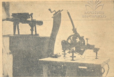
ინდუქტორი ინკლინატორი, რომელიც ზომავს მაგნიტის დახრის ბის კუთხეს. (იხ. ვ. ხუციშვილის წერტილი)
