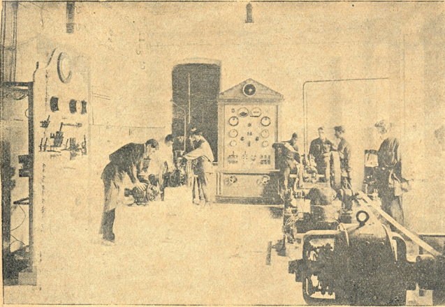
თბილისის ინდუტ. ტექნიკ. მანქანათა საცდელი ლაბარატორია.
