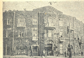
ნაძალადეში რკინის-გზელ მუშათა 4 სართულიანი სახლი, 57 ოთახით და კვეშ ხაეტების უნივერსალური მაღაზიით.
