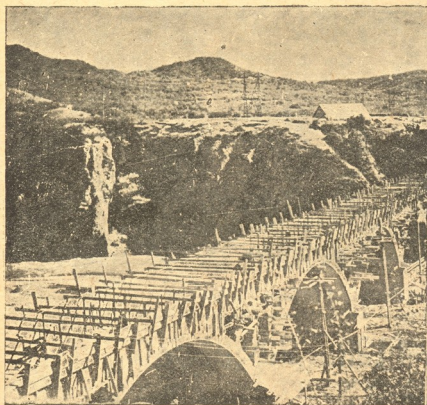
ნატახტარის წყალსადენი. ხიდი რომლის ქვეშაც გადის წყლის მილი, მთავარი მილი
