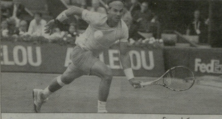
ნადალი რადიკალი
