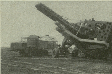
შემსლავრი ექსკავატორი „ერტ-801“ მშენებლობაზე.
