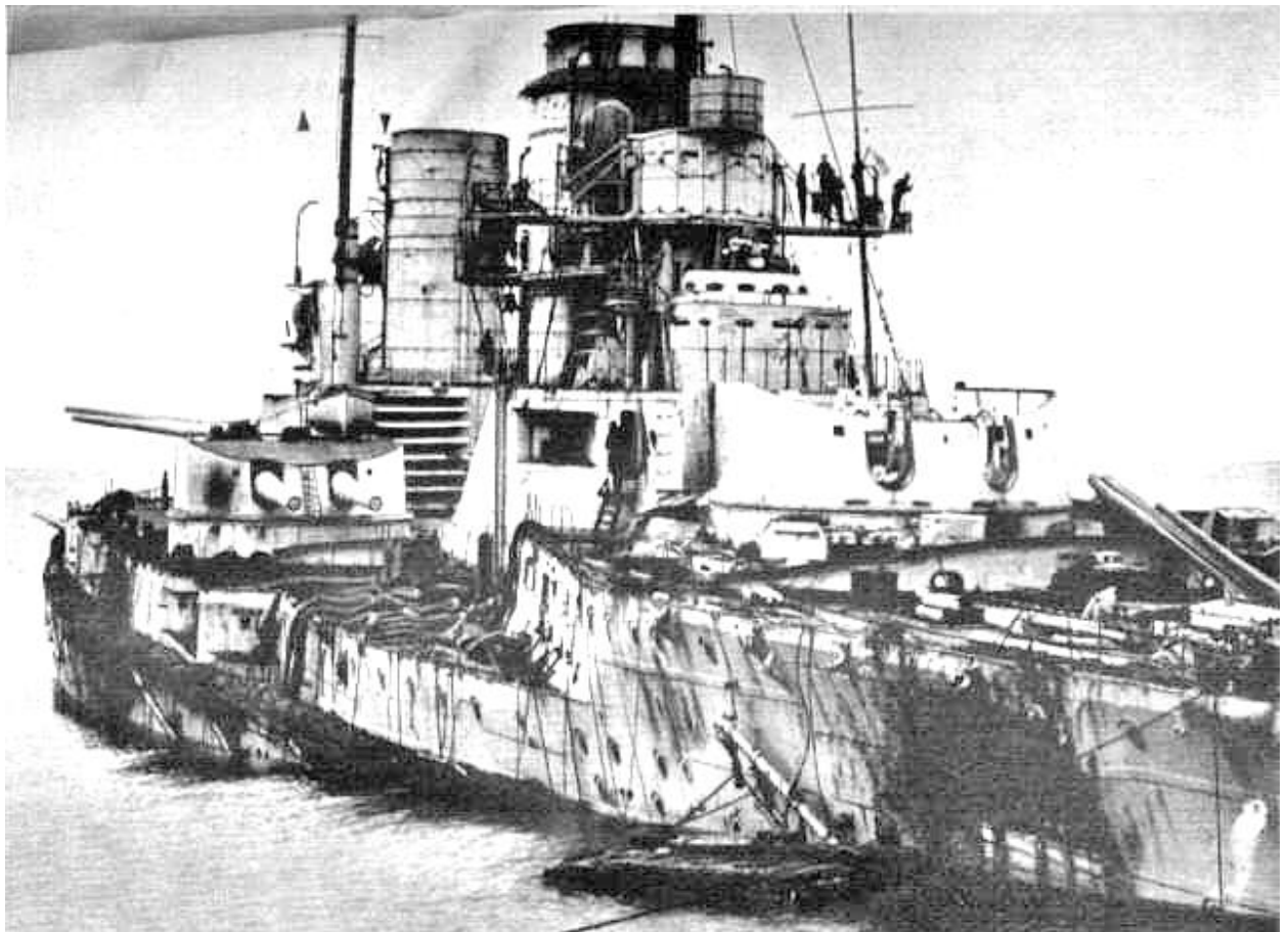
კრეისერი „ზაიდლიცი“ სკაგერაკის ბრძოლის შემდეგ
