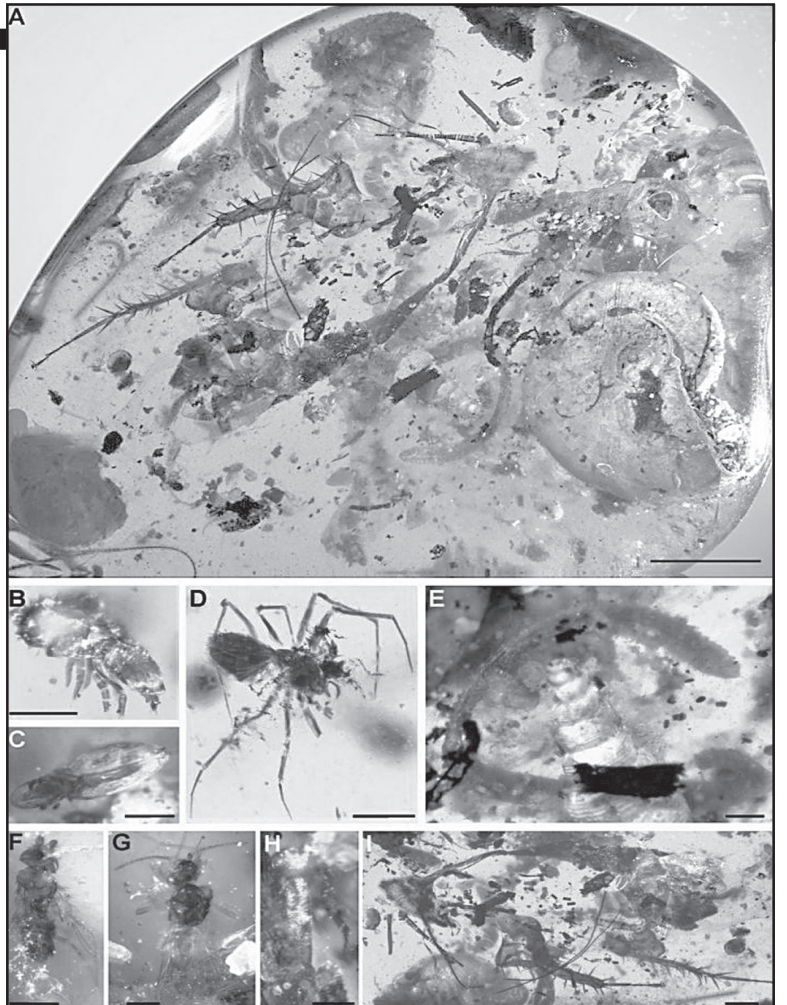
ნიჟარები. გაქვავებული ქარვა თანდათან ქვიშაქვის ქანებში დაფარა. სწორედ ამ გზით შემორჩნენ ეს უძველესი, განმარხებული არსებები ისტორიას
