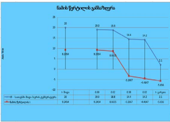
ნახ. 4.27. შემომფარგლავი კედლების გაანგარიშება
