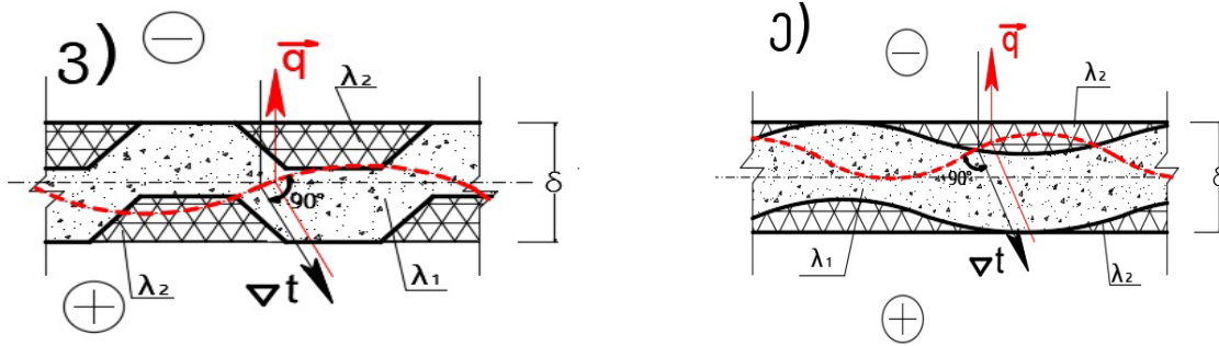
ნახ. 6.4. შემოთავაზებულ არაბრტყელზედაპირიან შრეებიან შემომფარგლავი კონსტრუქციის i - ურ კვეთში იზოთერმული ხაზის, ტემპერატურის გრადიენტის ვექტორის და სითბური ნაკადის ვექტორის მიმართულებები:
