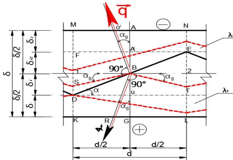
ნახ. 6.6. ორშრიანი შემომფარგლავი კონსტრუქცია
