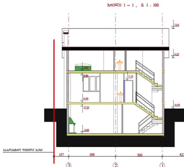
ნახ. 4.5. კრილი 1-1
