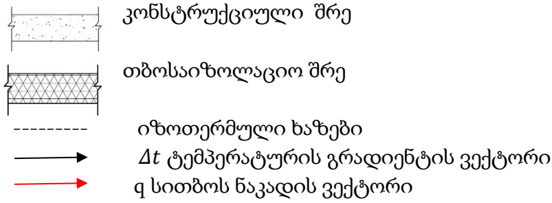
ნახ. 6.3 . ტემპერატურული გრადიენტის და სითბოს ნაკადის მიმართულებები შემომფარგლავ კონსტრუქციებში ბრტყელზედაპირიანი შრეებით: ა) ერთშრიანი, ბ) მრავალშრიანი
