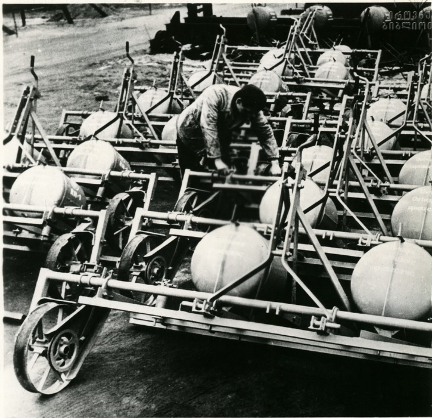
Разбрызгиватели жидкого аммиака, изготовляемые на заводе «Уния».
