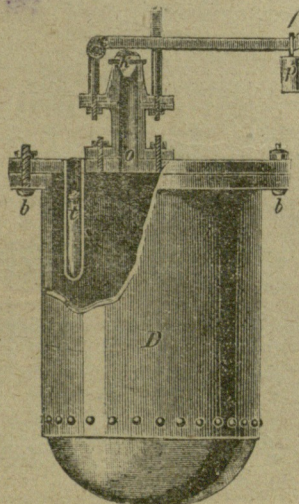
პაპინას ქვაბი.
