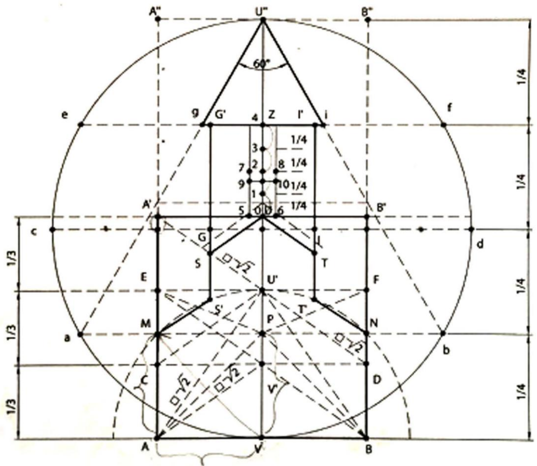
ნახ. N2 - სვეტიცხოვლის ტაძრის აღმოსავლეთ ფასადის სქემა
