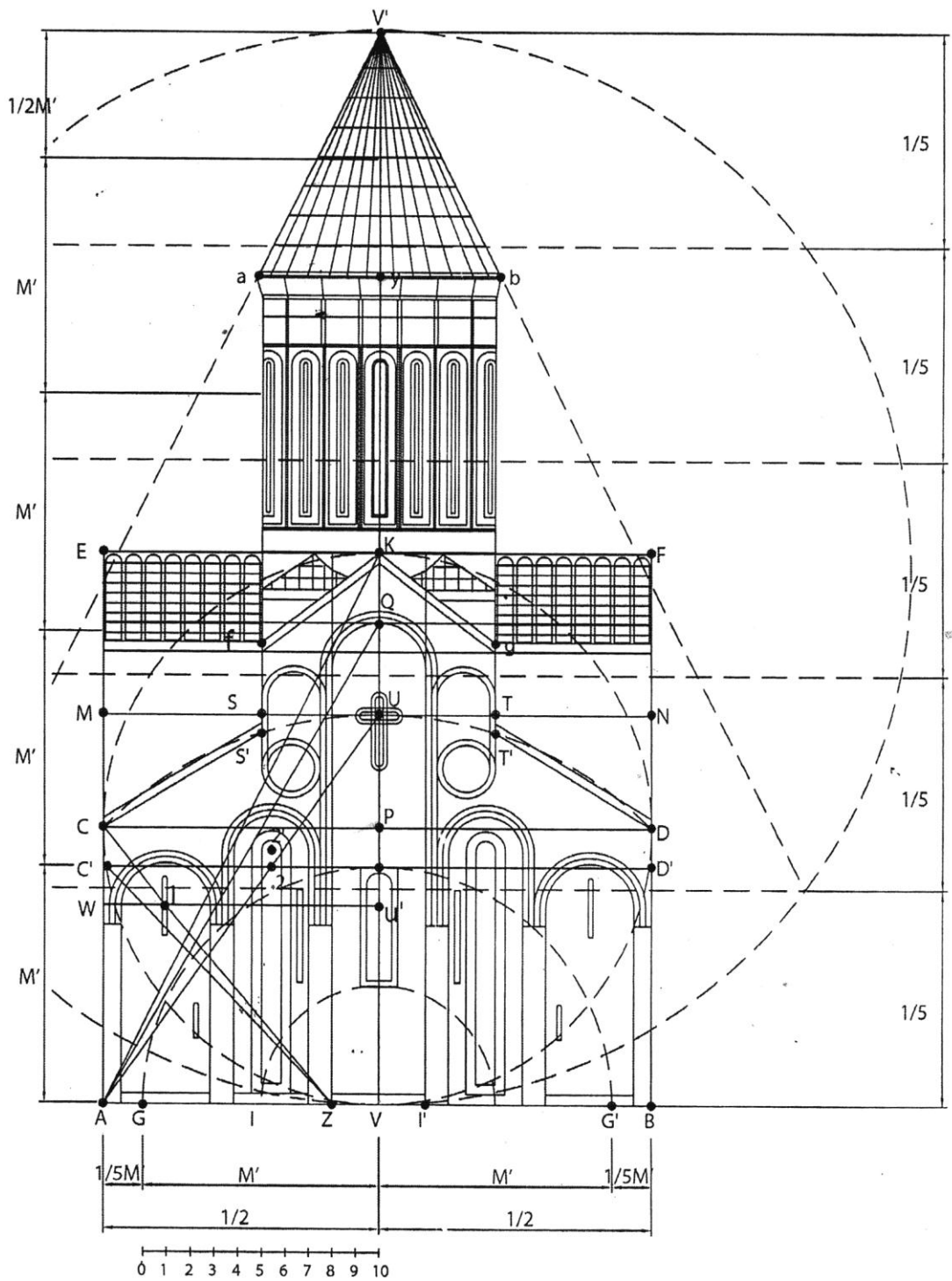
ნახ. N6 - ალავერდის ტაძრის ფასადის პროპორციულობის განსაზღვრა
