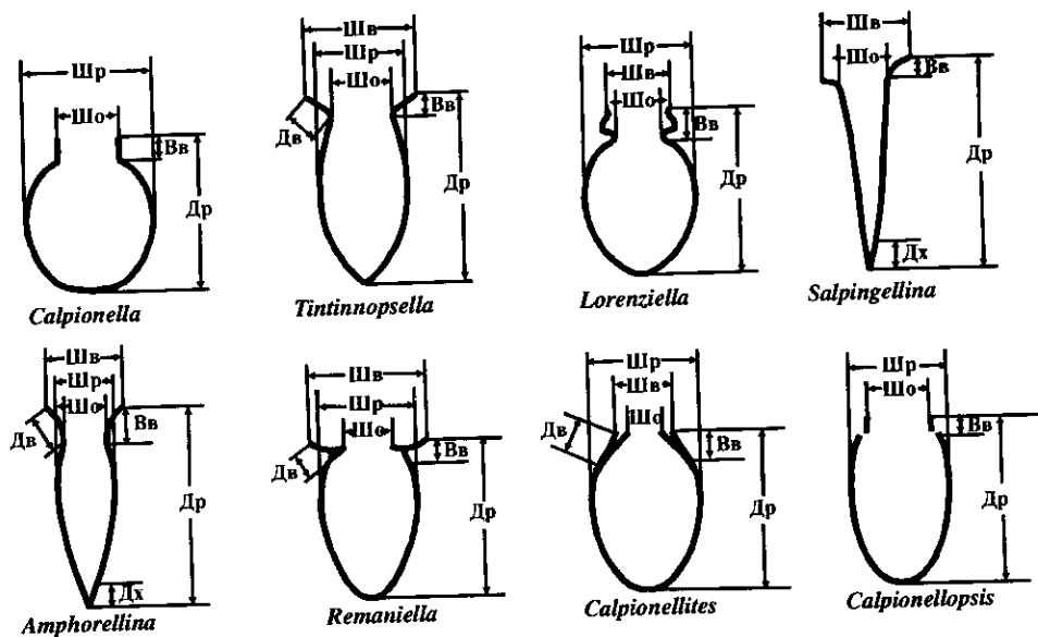
Рис. 8. Схемы строения раковин раннемеловых родов кальпионеллид.
