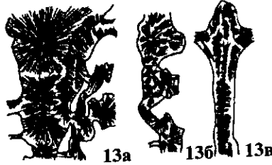
Рис. 13. а - простые склеродермиты, б - сложные, в - срединная темная линия
