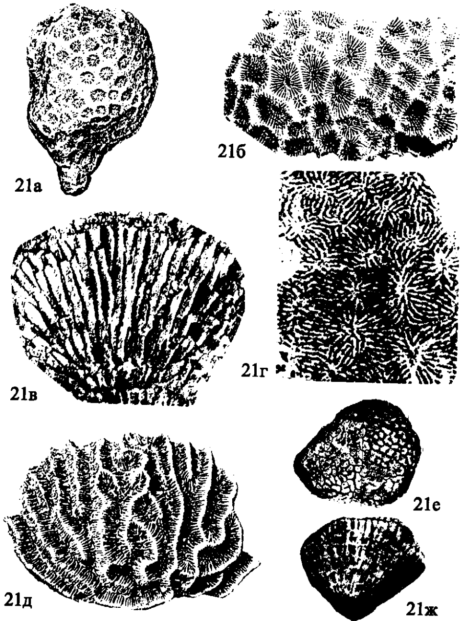
Рис. 21. Морфологические виды колоний: а - плокOIDная, б - периOIDная (сотовидная), в - фацилоидная (ветвистая), г - тамнастериOIDная, д - меандроидная, е, ж - гиднопороидная.
