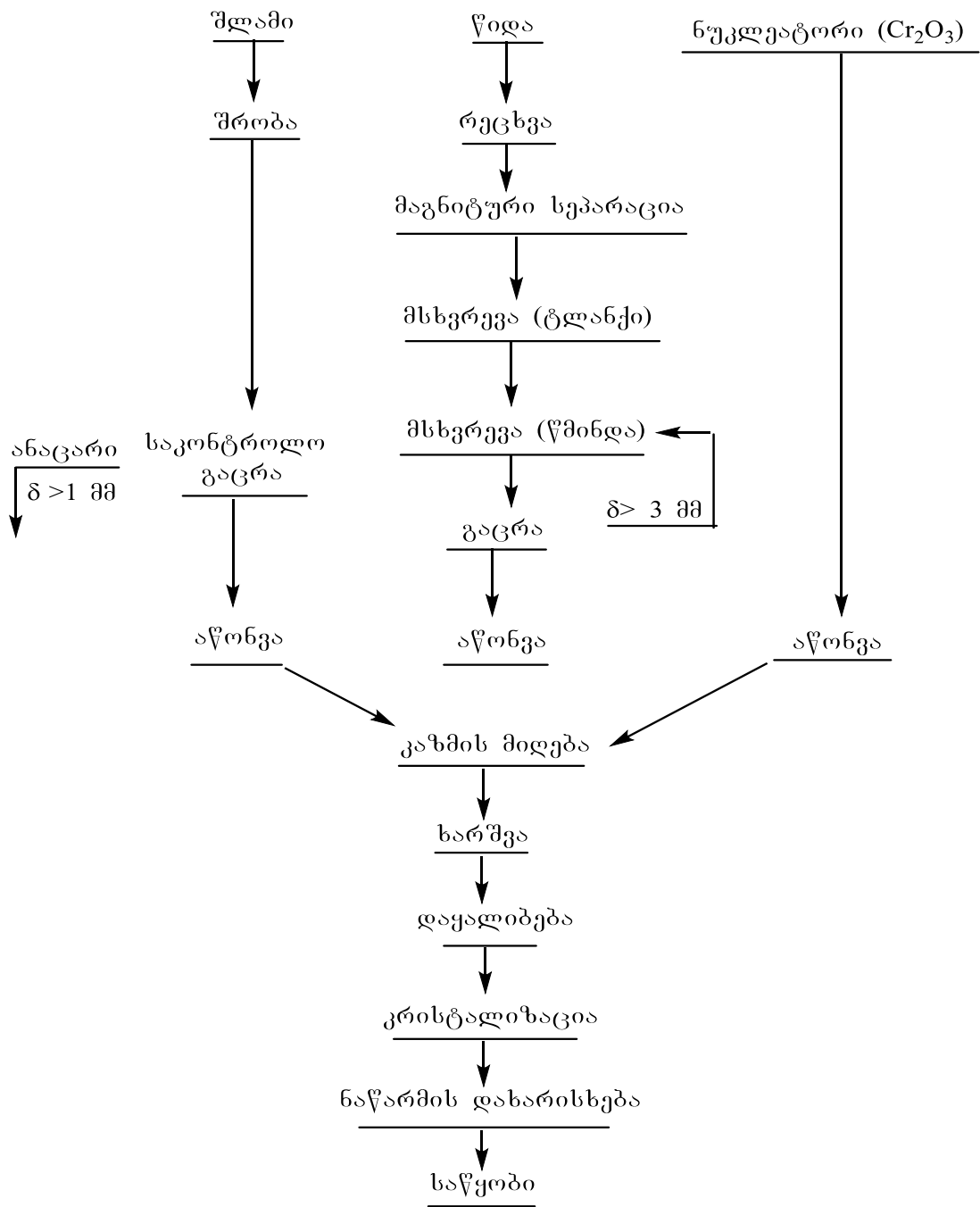
ნახაზი 10. „შლამი-წილა“ ნარევიდან ქვის სხმულის ნაწარმის მიღების რეკომენდირებული ტექნოლოგიური სქემა
