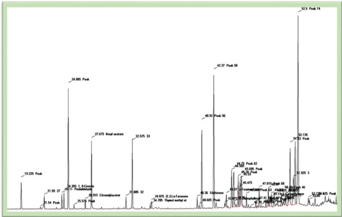
სურათი 25. ბადიანის ( Illicium verum ) ნაყოფის ეთერზეთის GC ქრომატოგრამა.
