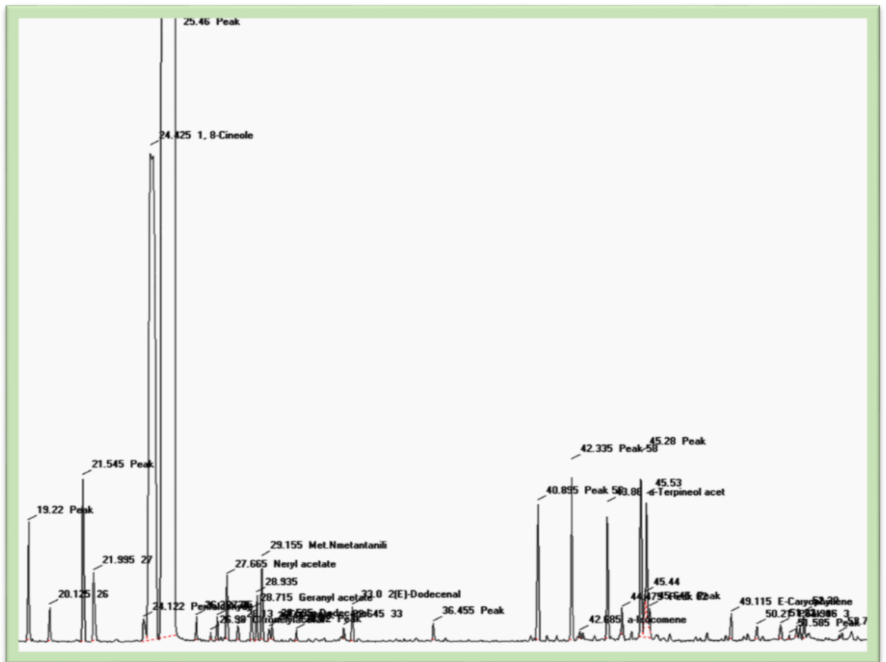
სურათი 24. Lindera communis ნაყოფის ეთერზეთის GC ქრომატოგრამა.
