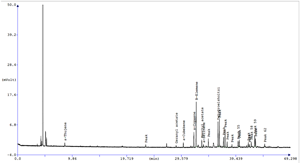
სურათი 23. ლეპტოსპერუმის ფოთლის ეთერზეთის GC ქრომატოგრამა.
