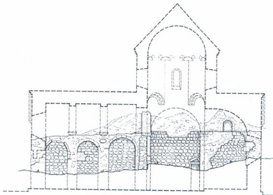
140. ისი, ქრილი წრდილოეთზე. გამოსაზა ნ. ბაგრატიონმა
