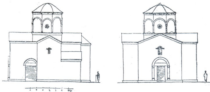
130. თელოვანის ჯვარიპატოსანი, საშრეთი და დასავლეთი ფასადები ვ. ცინცაძის მიხედვით
