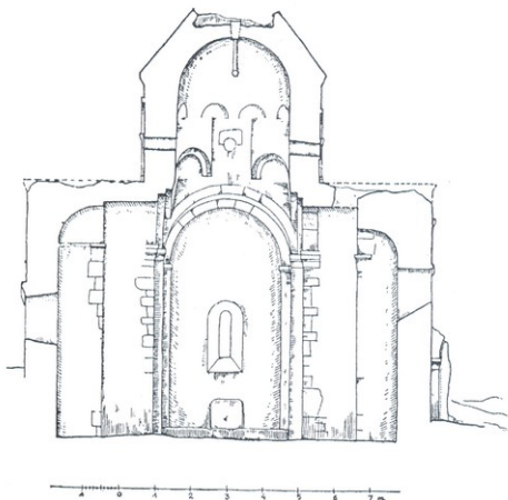
131. თელოვანის ჯვარიპატიოსანი, ქრილი აღმოსავლეთზე ვ. ცინცაძის მიხედვით
