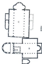
Fig. 6. Cimitile-Nola, Grab des hl. Felix (A), I. Kirche (B), Paulinus' Kirche (C) (Anlagen von 394-402)
