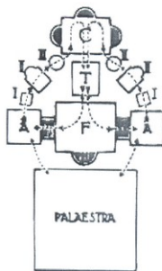
6. ანტიკური თერმების წყლის მიმოქცევის სქემა
