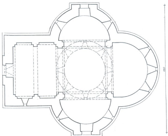
202. ჯვარზენის ტრიკონქი, გეგმა, აზომეს ც. დადიანიძემ და ლ. გიორგაძემ
