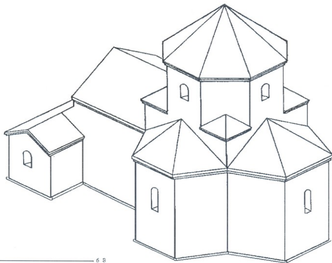
155. დორთ ქილისას ტრიკონქი. აქსონომეტრიული რეკონსტრუქცია
