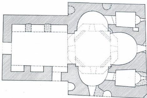
139. ისი, გეგმა, აზომა და გამოსაზა ნ. ბაგრატიონმა
