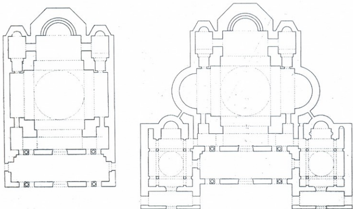
215-216. ათონის დიდი ლავრა, კათოლიკონი, მშენებლობის I და III ფაზები
