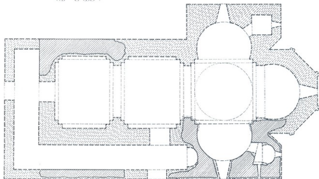
43. ზეგანის (ზაქი) ტრიკონქი, გეგმა. აზომა და გამოსაზა არქ. ნ. ბაგრატიონმა, 1966წ.
