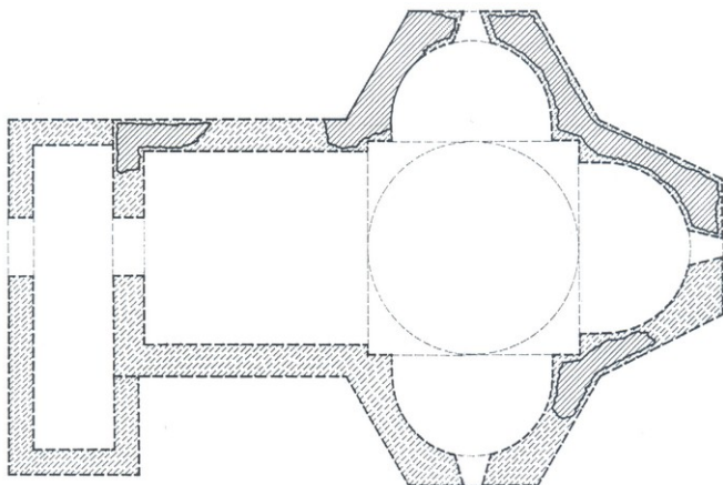
154. დორთ ქილისას ტრიკონქი. გეგმა. აზომა და გამობაზა ნ. ბაგრატიონმა
