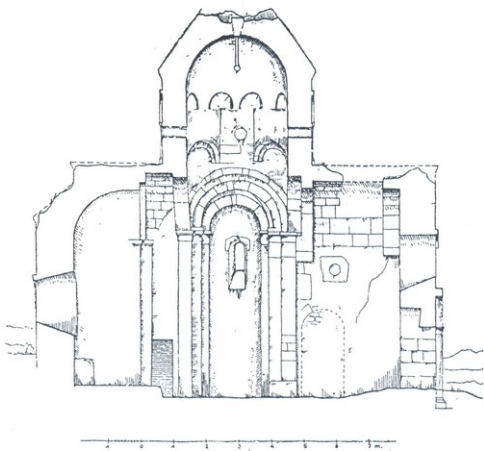
132. თელოვანის ჯვარიპატიოსანი, ქრილი სამხრეთზე ვ. ცინცაძის მიხედვით
