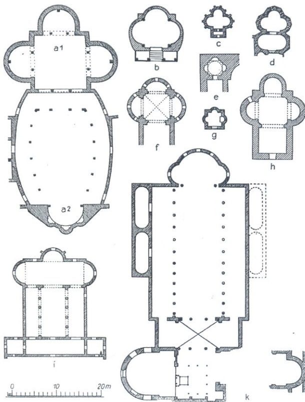
Abb. 5. Trichorische Bauten: a. Röm. Villa in Piazza Armerina (nr. 12); b. Mausoleum der Sabina, Sardos (nr. 39); c. Mausoleum, Pécs (nr. 27); d. Martyrium (?), Parenzo (nr. 26); e. Kirche (?), Sidi Mohammed el Gebiu (nr. 89); f. Memoria (?), Ptolemais (nr. 87); g. Baptisterium, Didyma (nr. 33); h. Kirche, Ed Dschumene (nr. 46); i. Basilika, Paramythia (nr. 38); k. Felixbasilika, Cimitile (nr. 8).
