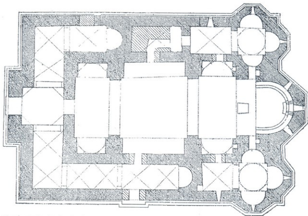
123. ვაჩნაძიანის ყველაწმინდა, გეგმა | სართულის დონეზე
