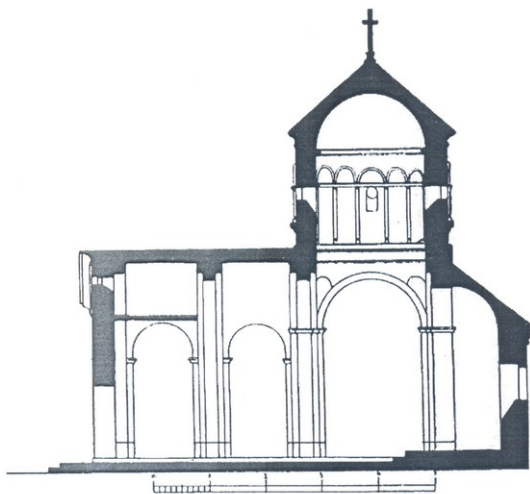
48. ზეგანი (ზაქი), ქრილი ჩრდილოეთზე ს. კლდიაშვილის მიხედვით, გამოცემული ექ. თაყაიშვილის მიერ
