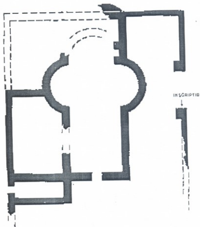
211. ჯალის მონასტერი, ტრიკონქი, გეგმა
