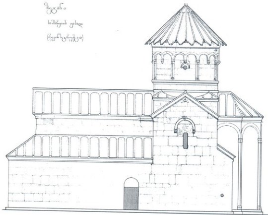
49. ზეგანი (ზაქი), სამხრეთი ფასადი, რეკონსტრუქცია არქ. ნ. ბაგრატიონის
