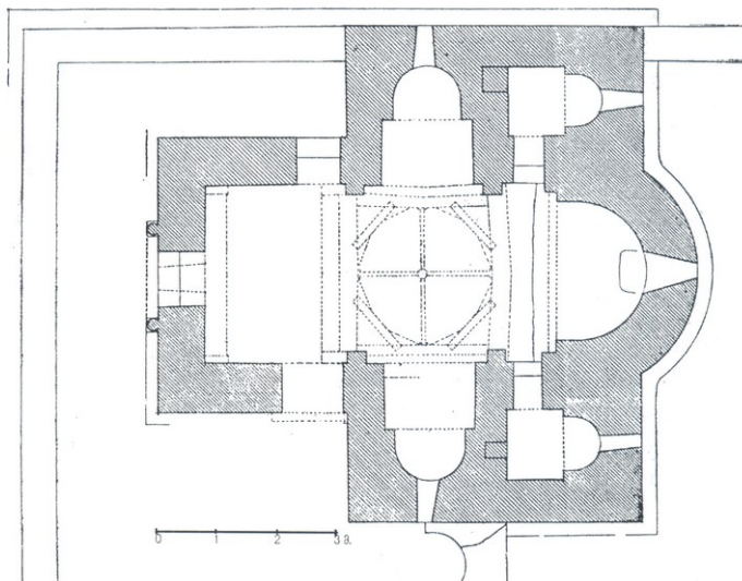
129. თელოვანის ჯვარიპატოსანი, გეგმა ვ. ცინცაძის მიხედვით
