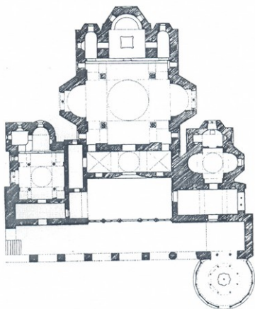
215-216. ათონის დიდი ლავრა, კათოლიკონი, მშენებლობის I და III ფაზები
