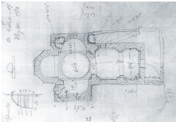
45. ზეგანი, გეგმა. კლდიაშვილის ნახაზი შესრულებული ძეგლის აზომვისას, 1907წ.
