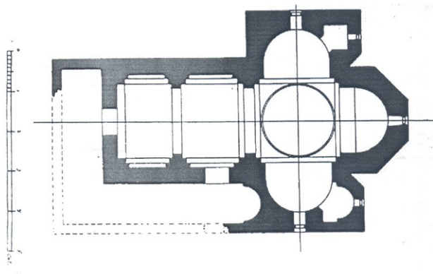
47. ზეგანი, გეგმა. კლდიაშვილის მიხედვით, გამოცემული ექ. თაყაიშვილის მიერ
