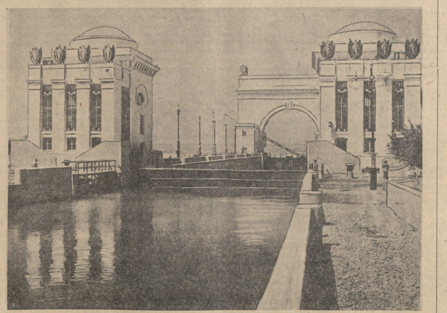
ვ. ი. ლენინის სახელობის ვოლგა-დონის სახანსო არხის № 13 რაბის ზემო სათავის სამართავი კოშკები (კარავის წყალხადავის მხარდა). ფოტო ს. კობაქიძის (საკ. დღეს) ფოტოქრონიკა.
