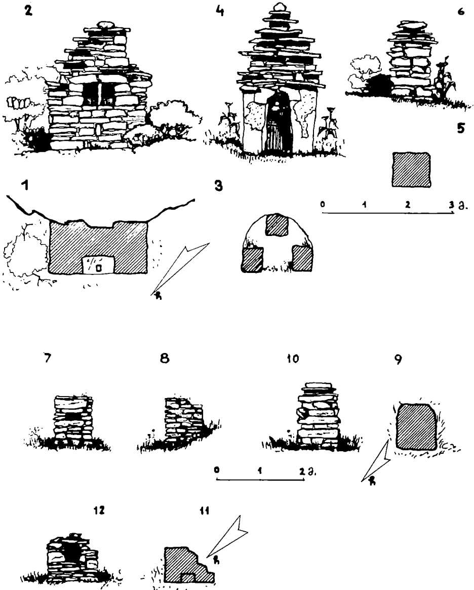
სოფ. ქალისოფელი. იახსრის წვარის კომპლექსი, 1962 წ. თაბარის კოშკი—1. გეგმა, 2. ფასადი; საზარე კოშკი—3. გეგმა, 4. ფასადი; დობილთ კოშკი—5. გეგმა, 6. ფასადი; სასანთლე კოშკი—7. ფასადი, 8. გვერდხედი; სასანთლე კოშკი—9. გეგმა, 10. ფასადი; დობილთ კოშკი—11. გეგმა, 12. ფასადი.
