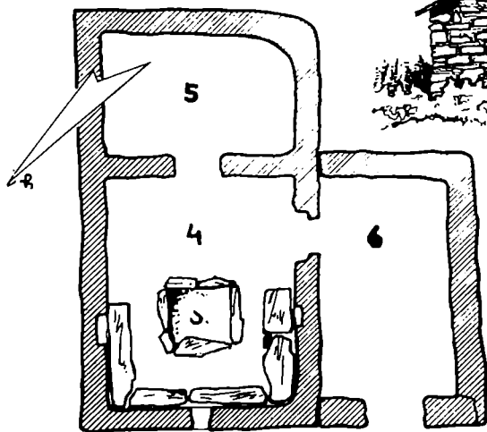
სოფ. ქალისოფელი, იახსრის წყარის კომპლექსი, 1962 წ. სიქეაბე — 1. გეგმა, 2. ფასადი, 3. კრილი (ა. კულა), დარბაზი, გეგმა — 4 დარბაზი (ა. კერა), 5. საკოდე, 6. საბერო, 7. ფასადი.
