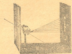
სპექტროსკოპი.
