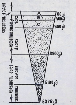
დედამიწის აგებულების სქემა.
