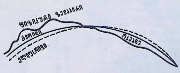
დედამიწის ფორმისა ზედაპირის ბოლოდის და პლანეტოიდის ურთიერთ დამოკიდებულების სხემა.
