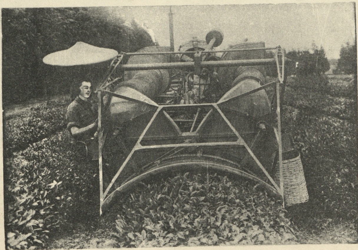
ტექნიკურ მეცნიერებათა კანდიდატის შალვა კერესელიძის და კონსტრუქტორთა ჯგუფის მიერ ახლად აგებული ჩაის მკრეფავი მანქანა, რომელმაც სახელმწიფო გამოცდა უკვე ჩააბარა და ჩვენს სახელმწიფო სტახანოველებთან ერთად შეუდგა ჩაის კრეფის გეგმის გადაჭარბებით შესრულებას...
