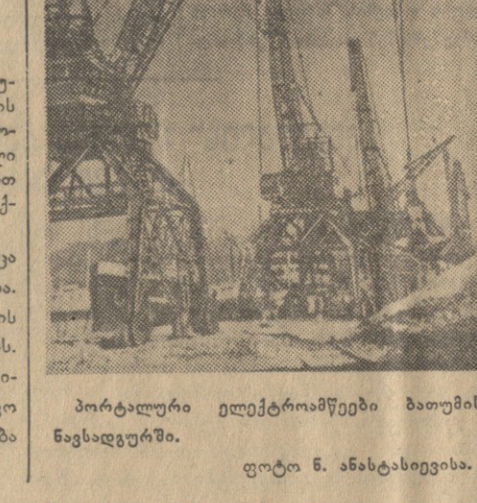
პორტალური ელექტრომწეობი ბათუმის ნავსადგურში.
