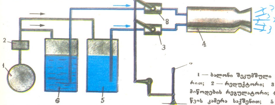
სითხიანი რაკეტული ძრავის სქემა
